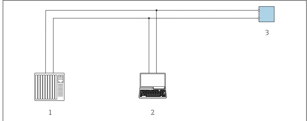
图 32 通过 Modbus RS485 通信进行远程操作 (有源信号)
