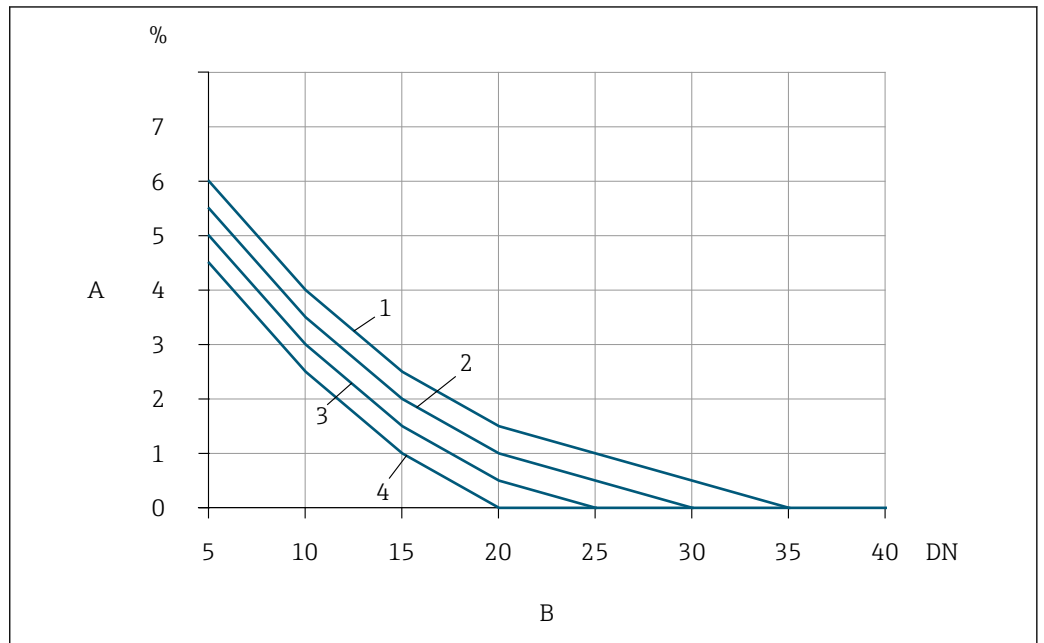
10 未安装流量调节器时可能存在的附加测量误差，与干扰因素和前管段类型相关
