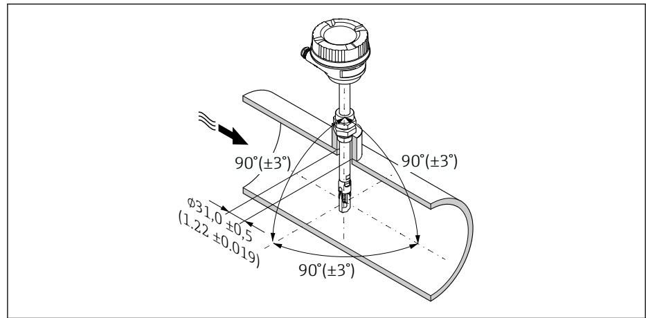
图 16 尺寸单位: mm (in)
