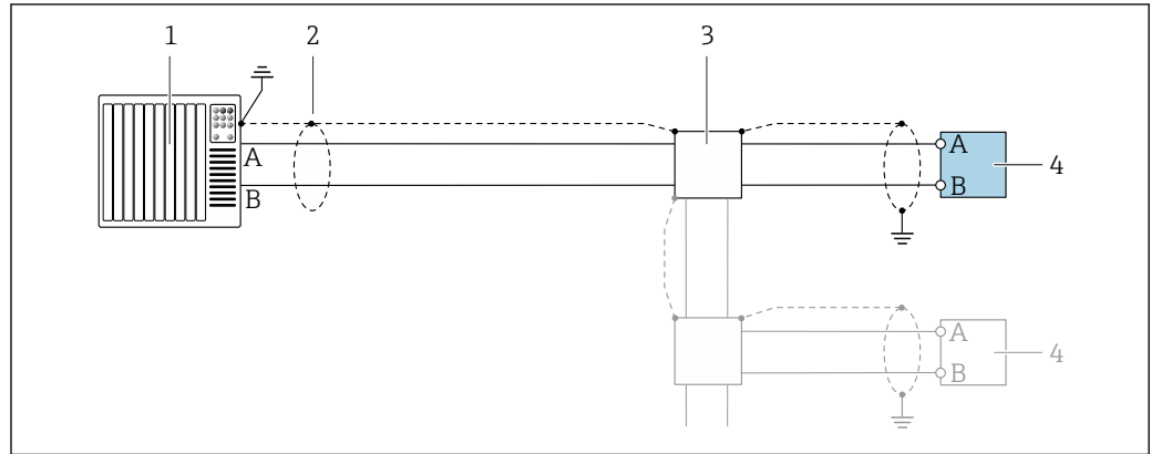
图 20 接线实例：Modbus RS485，非危险区和防爆 2 区；Cl. I, Div. 2 防爆场合
