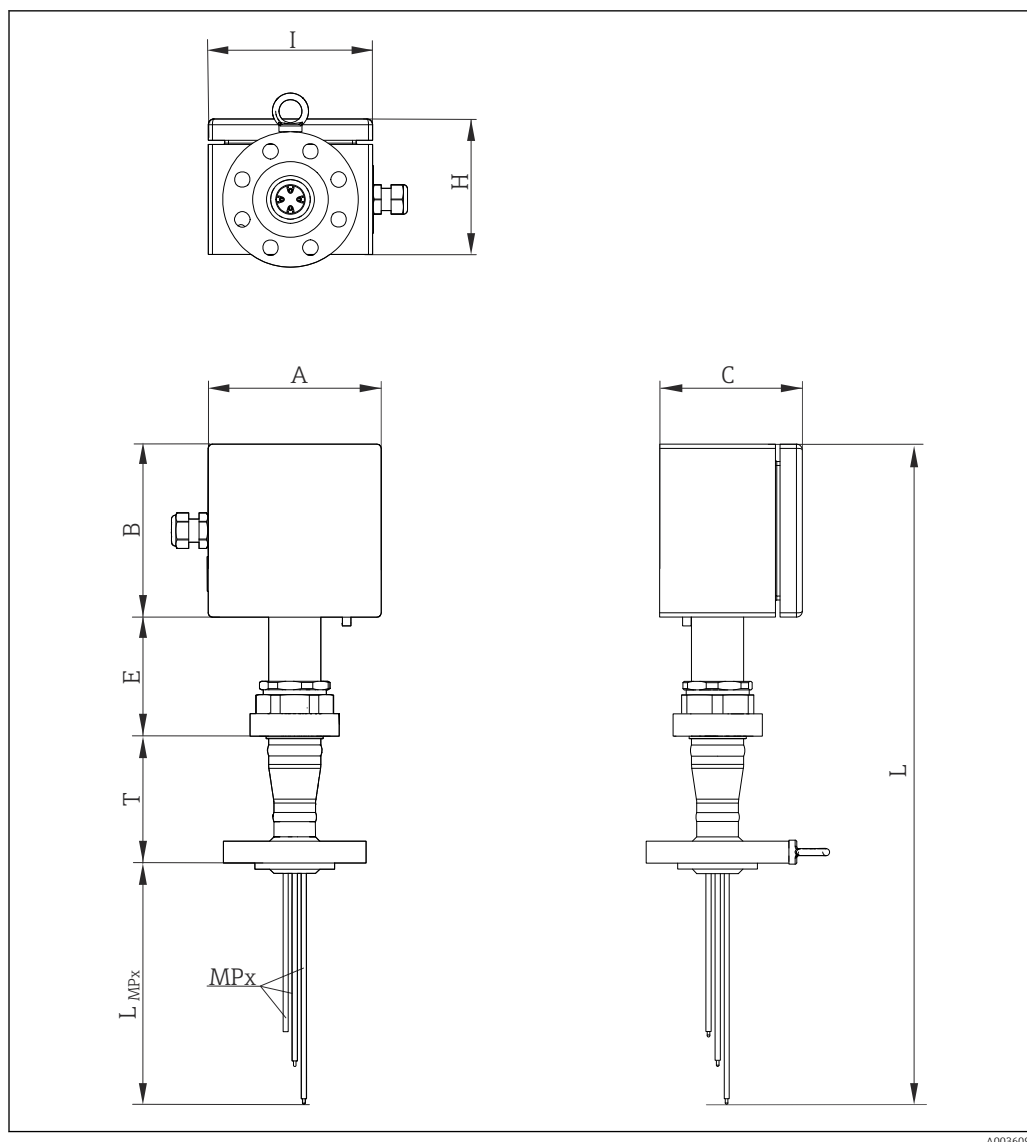
9 Diseño de la sonda de temperatura multipunto modular, con cuello para soporte tubular. Todas las medidas están expresadas en mm (in)
