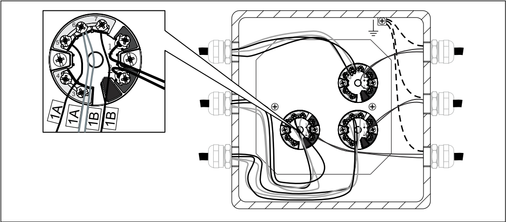
5 Transmisor para cabezal montado y cableado. Ejemplo de marcado de los cables de un sensor interno con 2 x TC
