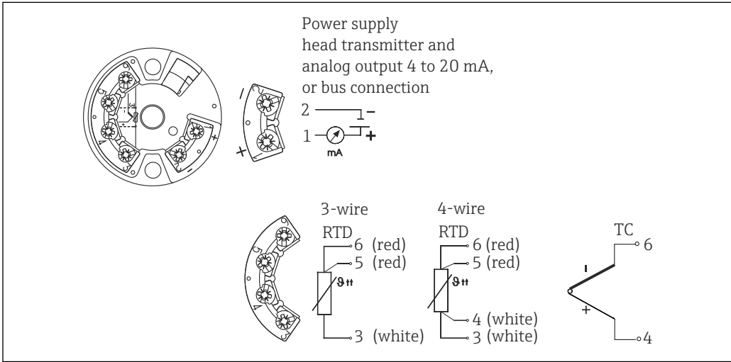
3 Diagrama de conexionado de los transmisores para cabezal con entrada para sensores única (TMT18x)
