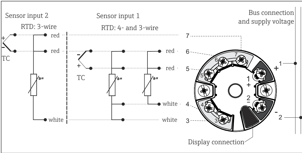
2 Diagrama de conexionado de los transmisores para cabezal con entrada para sensores dual (TMT8x)
