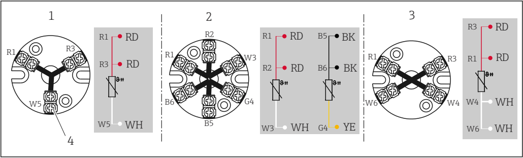
2 安装有端子接线块
