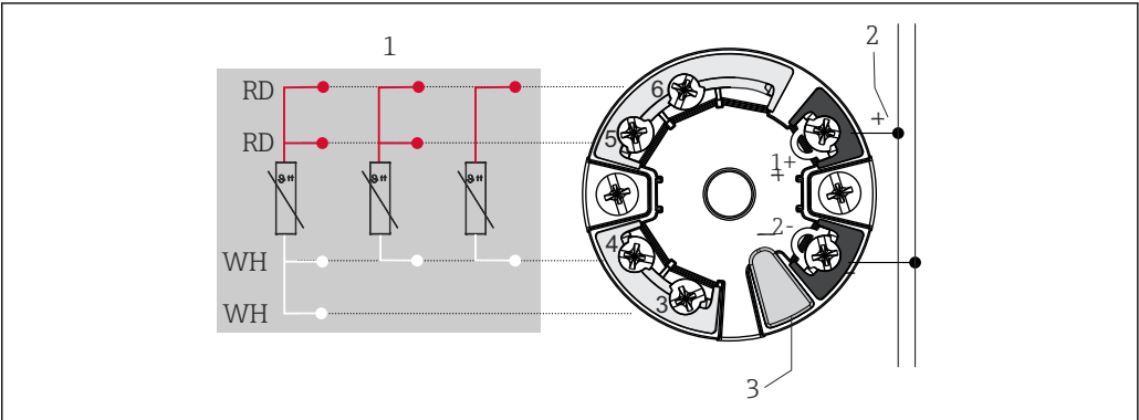
4 TMT7x 或 TMT31 模块化温度变送器 (单输入通道)
