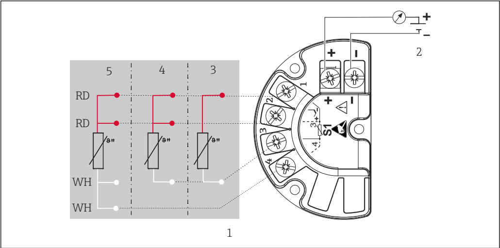
图 7 TMT142B 现场型温度变送器（单输入通道）
