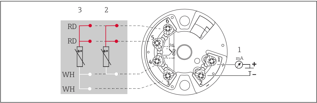
3 TMT18x 模块化变送器 (单路传感器输入)
