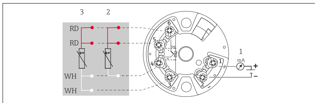
3 Transmetteur monté en tête TMT18x (une entrée capteur)
