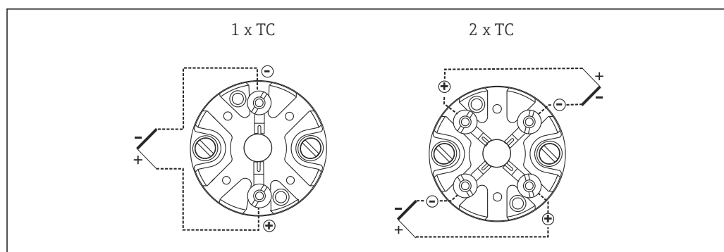
8 Bornier de raccordement monté
