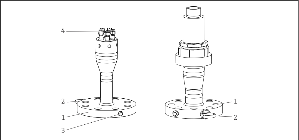
11 Bride en tant que raccord process
