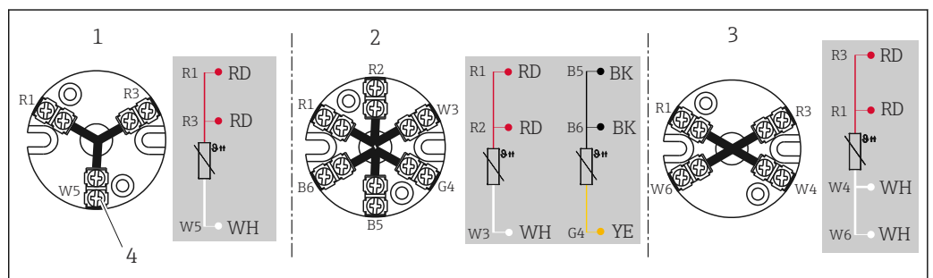
2 Bornier de raccordement monté
