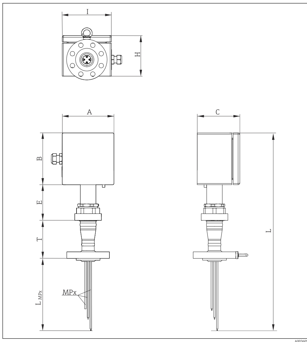
10 Construction du capteur de température multipoint modulaire, avec tube prolongateur. Toutes les dimensions en mm (in)
