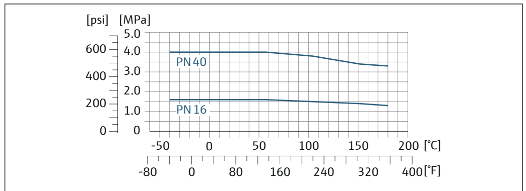
図 39 フランジ材質 1.4404/SUS F316L 相当/SUS F316 相当
