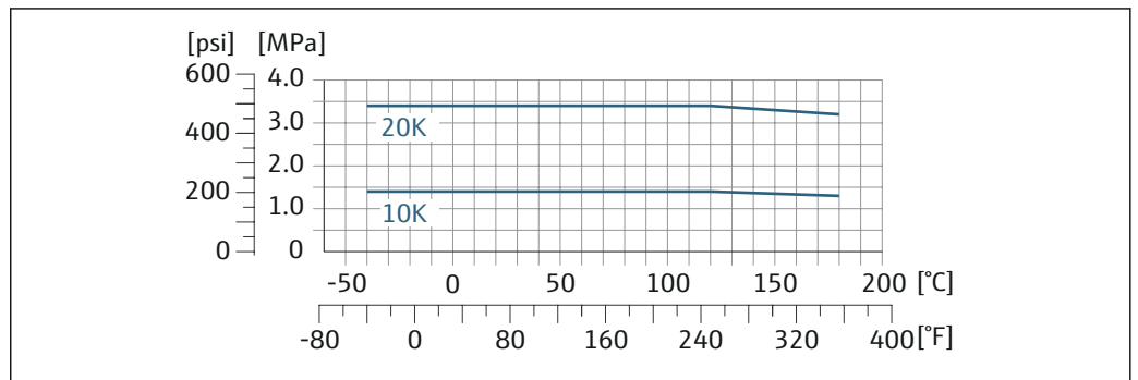
図 40 フランジ材質 1.4404/SUS F316L 相当/SUS F316 相当
