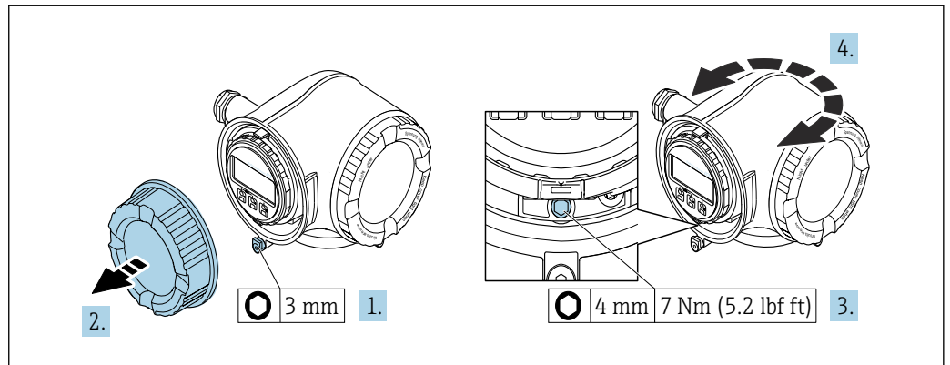
図 16 非防爆ハウジング
