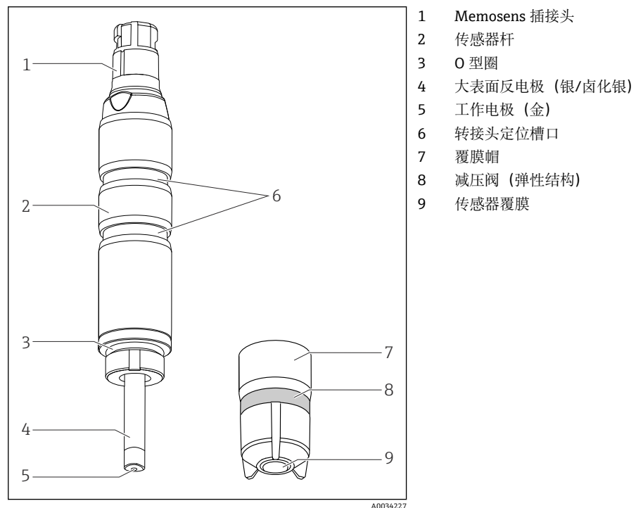
图 1 传感器结构
