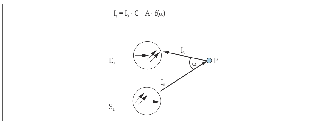
7 Princípio do método de luz retrodifusa
