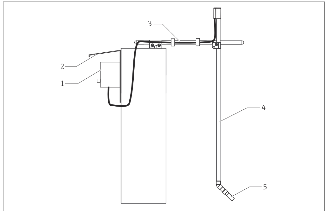
9 Sistema de medição com conjunto de imersão (exemplo)
