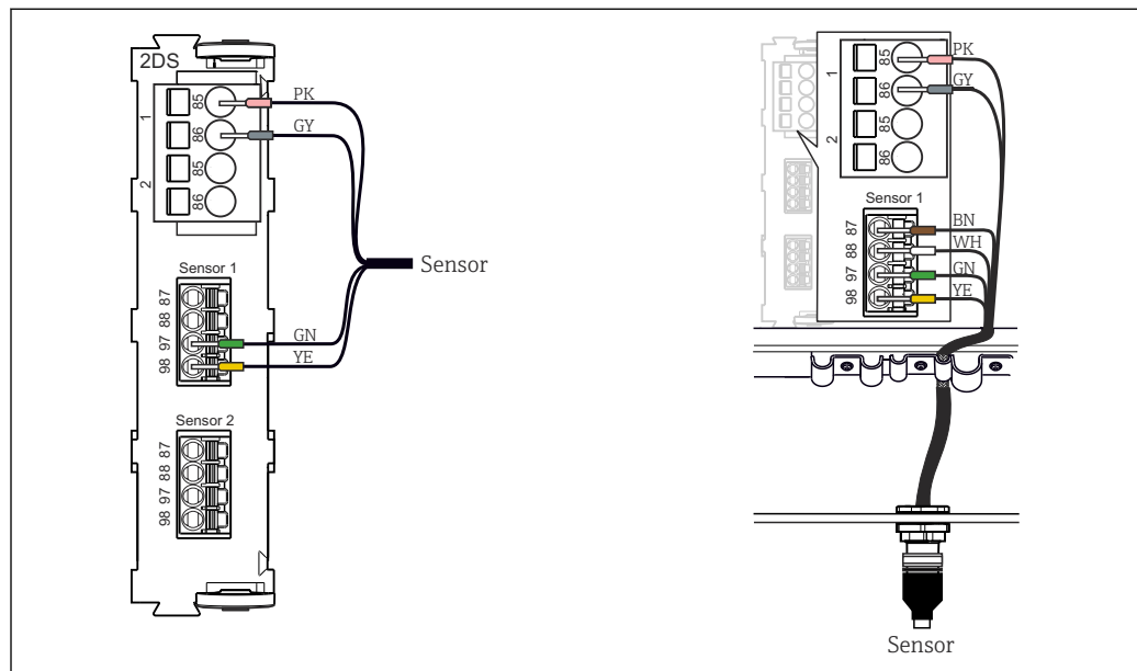
13 Conexão do sensor à entrada do sensor (esquerda) ou através do conector M12 (direita)
