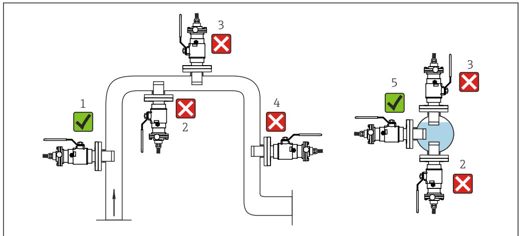
19 Orientações e posições (com conjunto retrátil CUA451)
