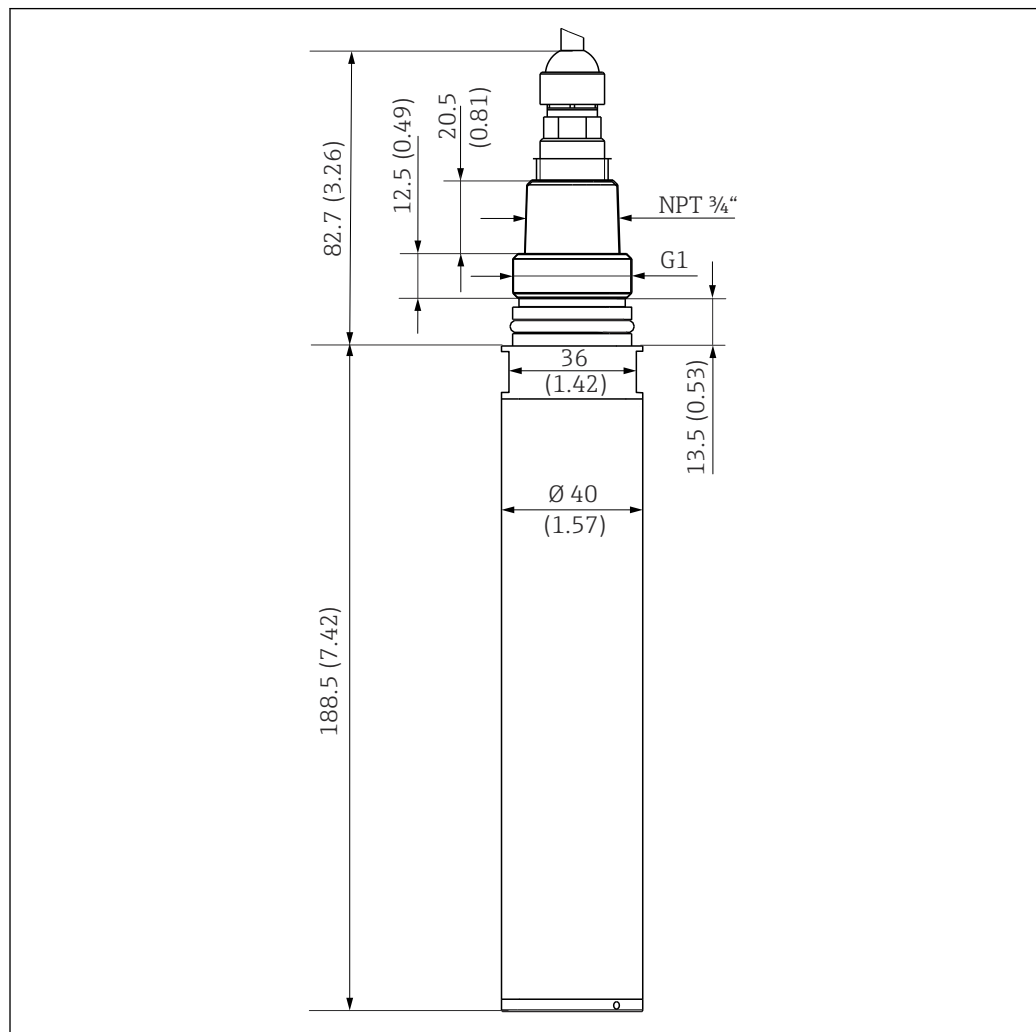
20 Dimensões . Unidade de engenharia: mm (pol.)
