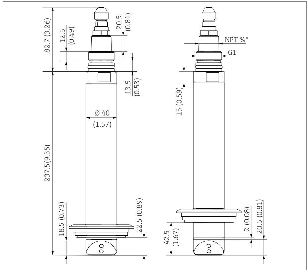
21 Dimensões do sensor de aço inoxidável com conexão Varivent padrão (esquerda) e eixo estendido (direita). Dimensões: mm (pol.)
