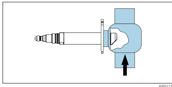
17 Instalação com conexão Varivent com haste estendida
