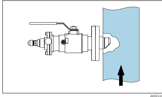
11 Instalação com conjunto retrátil CUA451
