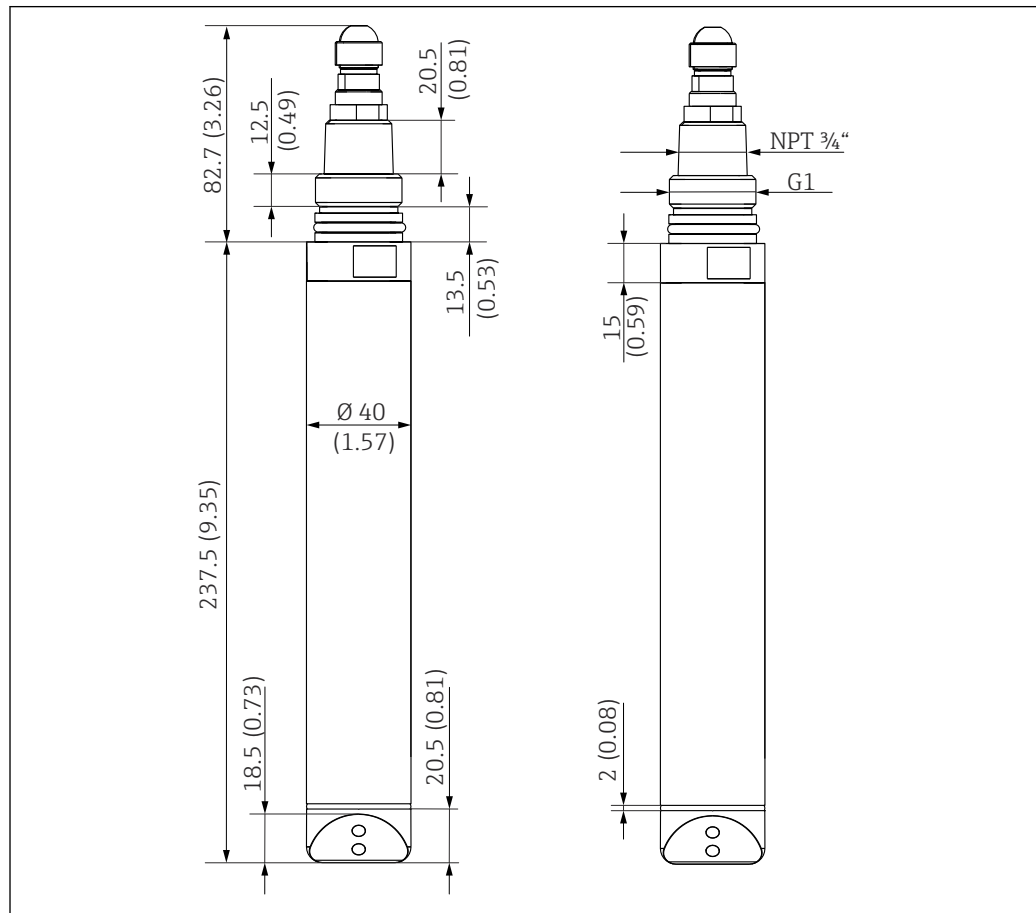
19 Dimensões do sensor de plástico. Dimensões: mm (pol.)
