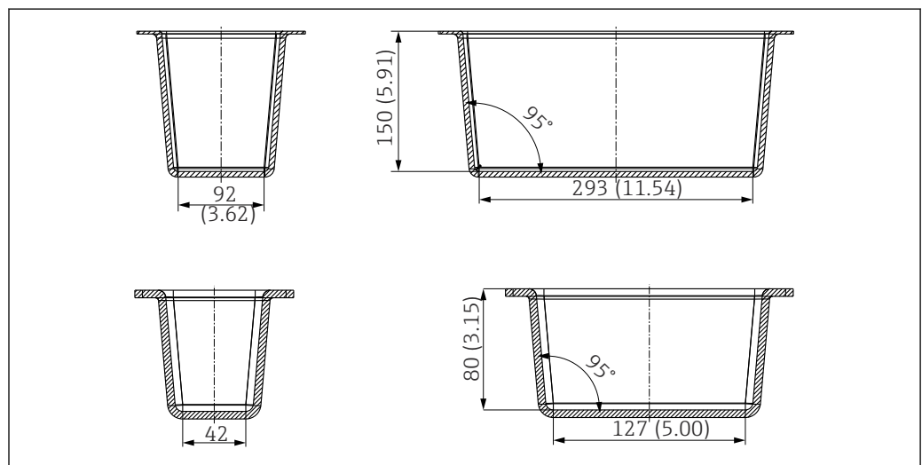
6 Recipiente de calibração grande (topo) e recipiente de calibração pequeno (base). Unidade de engenharia: mm (pol.)
