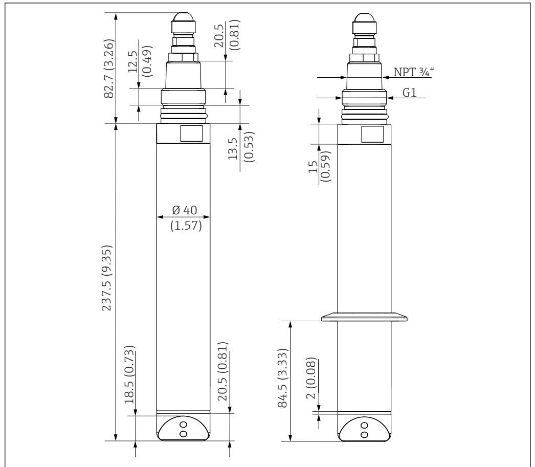
20 Dimensões do sensor de aço inoxidável e sensor de aço inoxidável com conexão de braçadeira (direita). Dimensões: mm (pol.)
