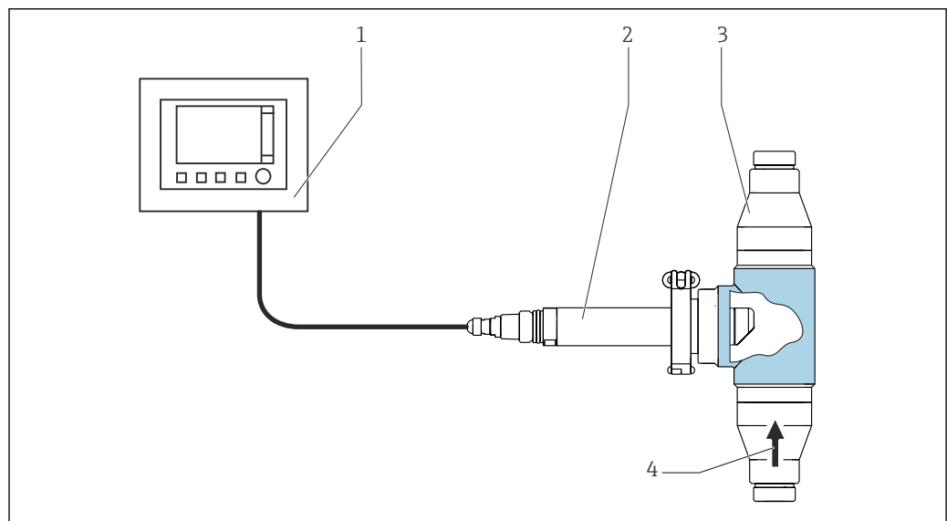
2 Exemplo de sistema de medição com conjunto de vazão CUA252, para sensor de aço inoxidável
