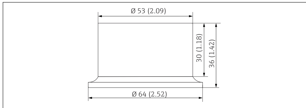
24 Adaptador soldado. Dimensões: mm (pol.)
