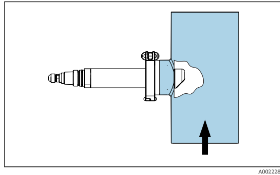
15 Instalação com conjunto de vazão CUA262
