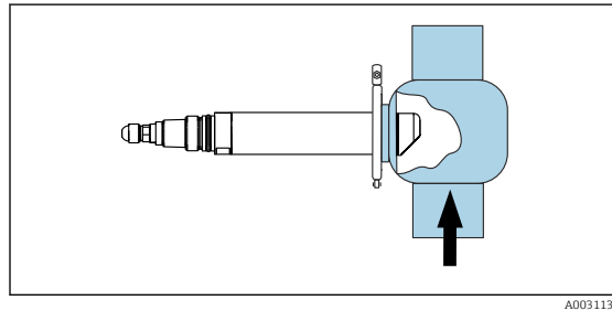
16 Instalação com conexão padrão Varivent
