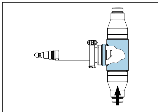
14 Instalação com conjunto de vazão CUA252
