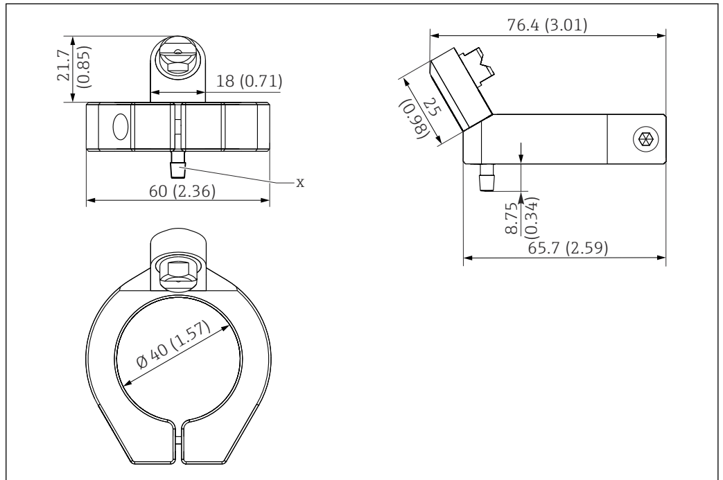
26 Limpeza por ar comprimido para sensores de aço inoxidável. Dimensões: mm (pol.)
