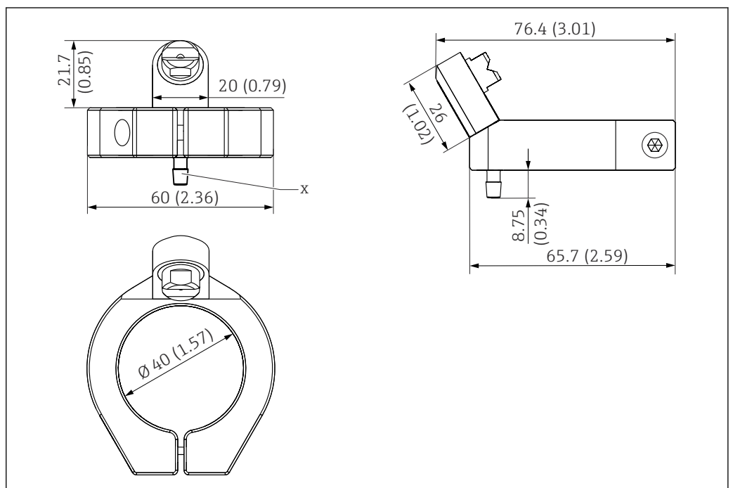
27 Limpeza por ar comprimido para sensor de plástico. Dimensões: mm (pol.)
