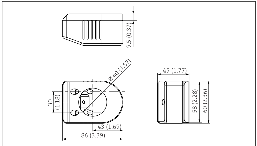
23 Referência de estado sólido Calkit CUS52D. Unidade: mm (pol.)
