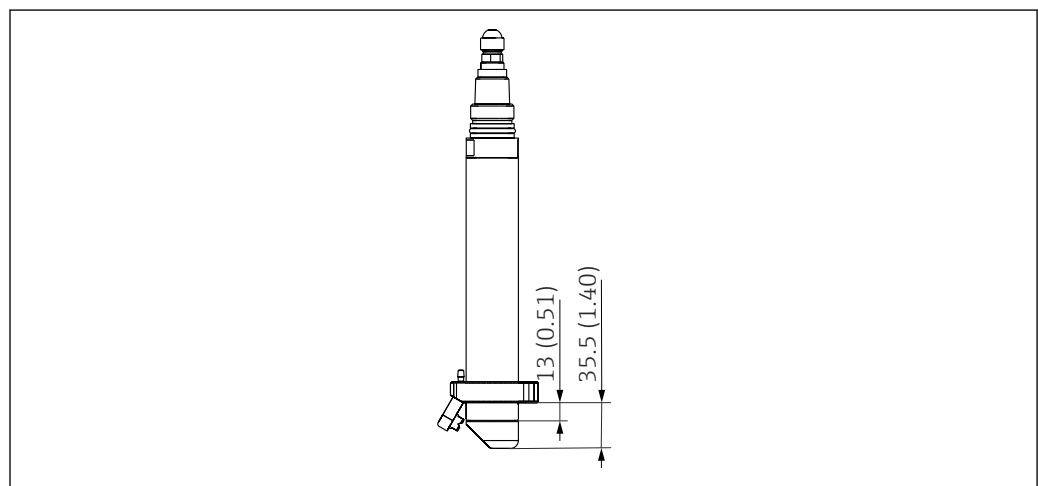
22 Dimensões do sensor com limpeza de ar comprimido. Dimensões: mm (pol.)
