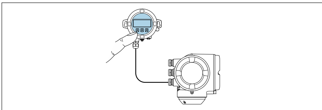
図 33 リモートディスプレイと操作モジュール DKX001 を使用した操作
