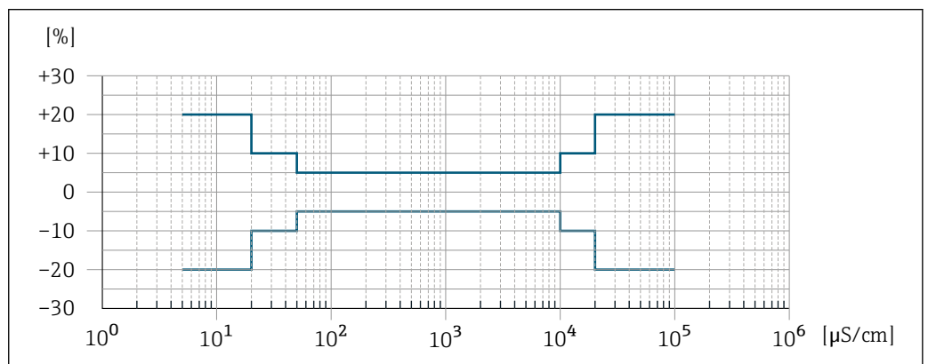
図 31 測定誤差 (オプション:「校正された導電率測定」のオーダーコード、オプション CW)
