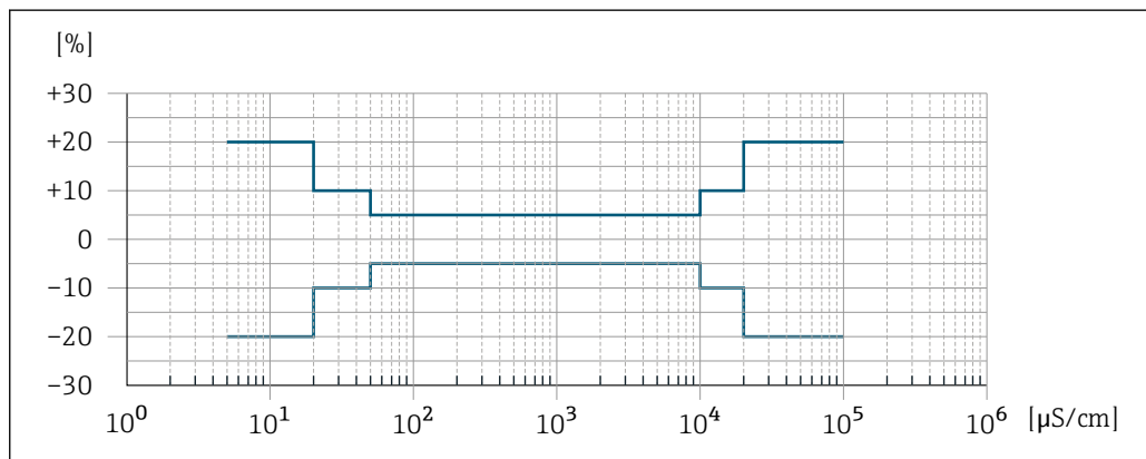
図 32 測定誤差 (オプション: 「校正された導電率測定」のオーダーコード、オプション CW) A0047944
