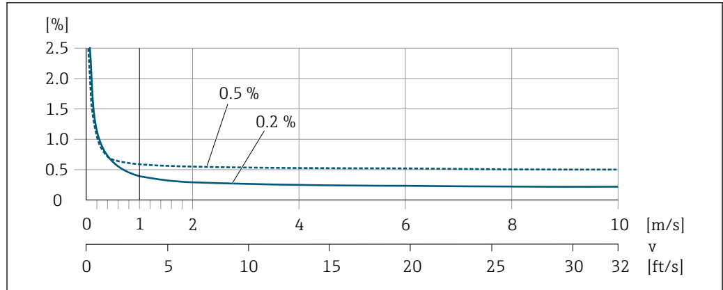
図 29 最大測定誤差 (%) o.r.
