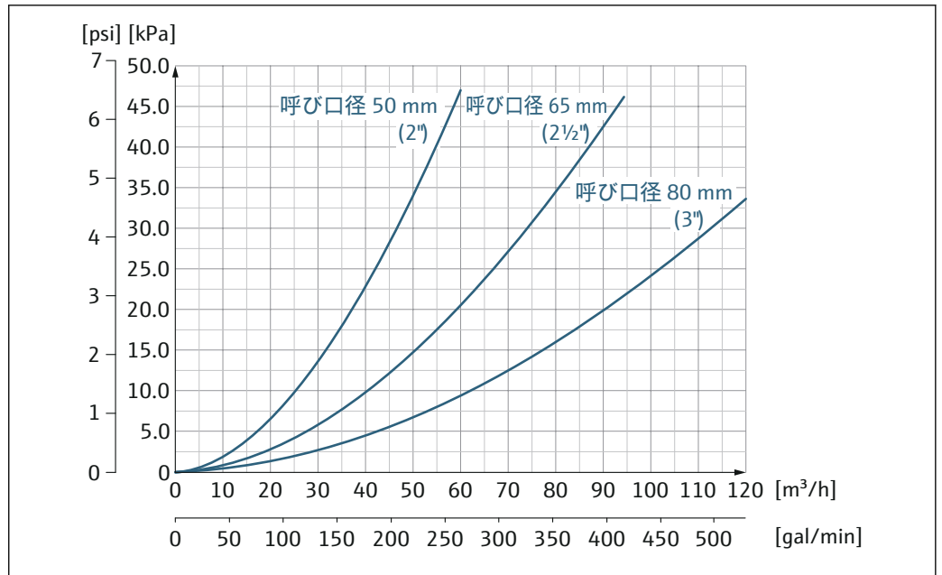
33 呼び口径 50～80 mm (2～3") の圧力損失：「設計」のオーダーコード、オプション C「固定フランジ、縮小計測チューブ、0x呼び口径 上流側/下流側直管長」の場合
