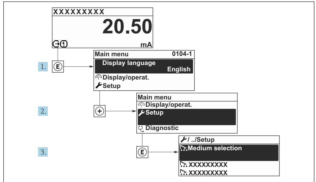
図 24 現場表示器の表示例
