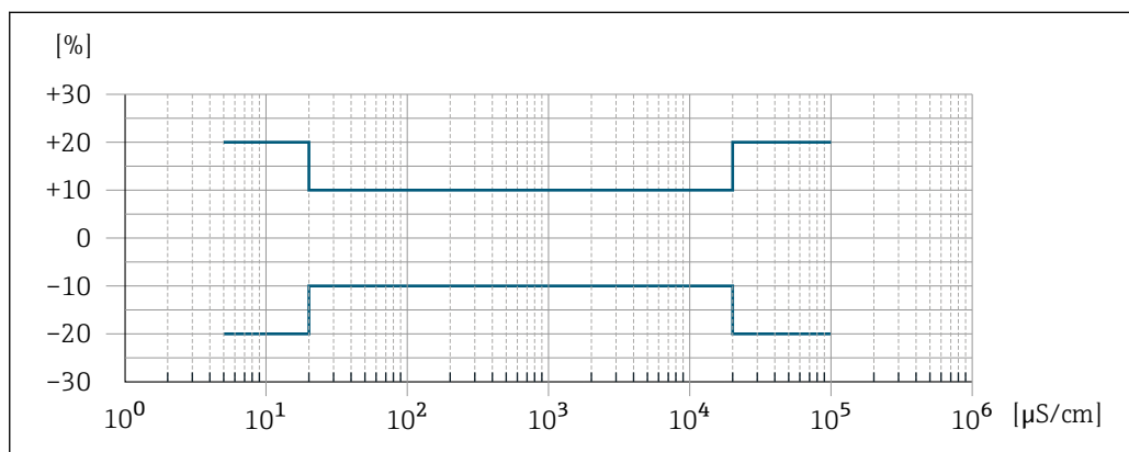
図 31 測定誤差 (標準) A0042279
