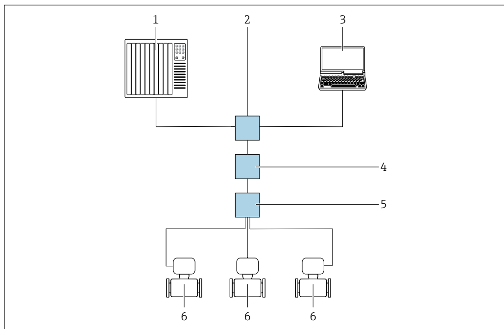
図 20 APL ネットワーク経由のリモート操作オプション
