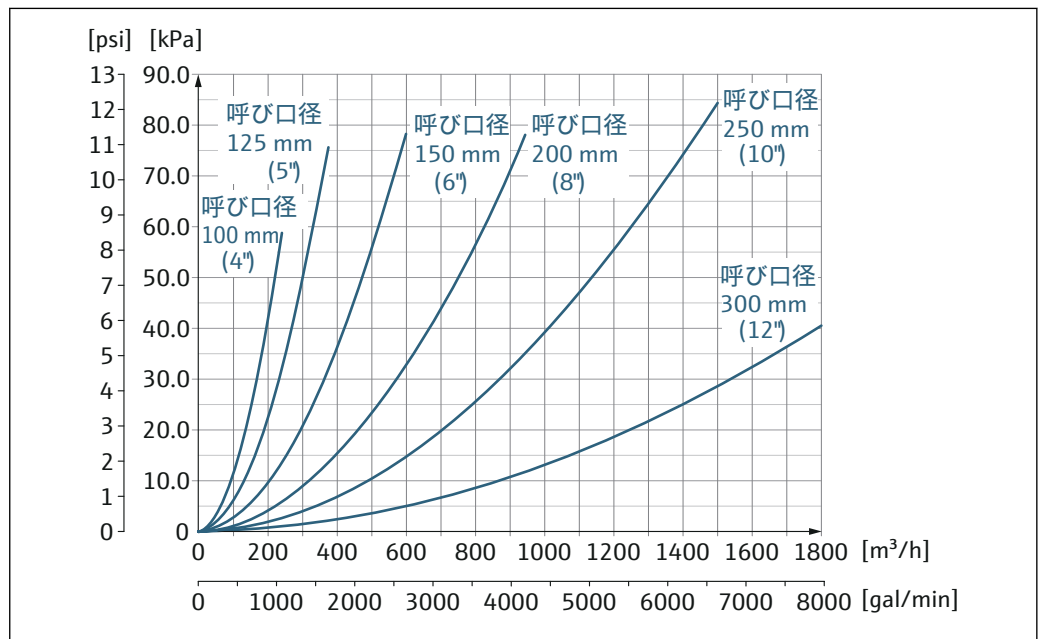
34 呼び口径 100～300 mm (4～12") の圧力損失：「設計」のオーダーコード、オプション C「固定フランジ、縮小計測チューブ、0x呼び口径 上流側/下流側直管長」の場合
