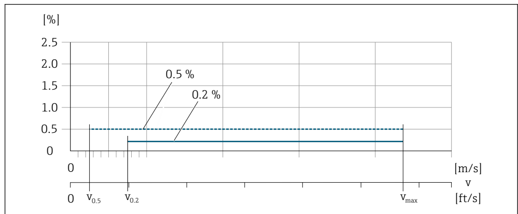
図 30 フラットスペック (%) o.r.
