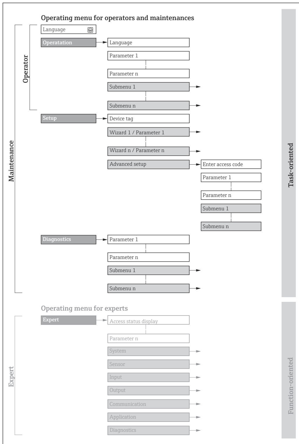
16 操作メニューの概要構成
