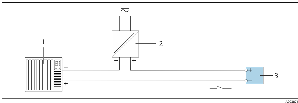
図 18 リレー出力（パッシブ）の接続例
