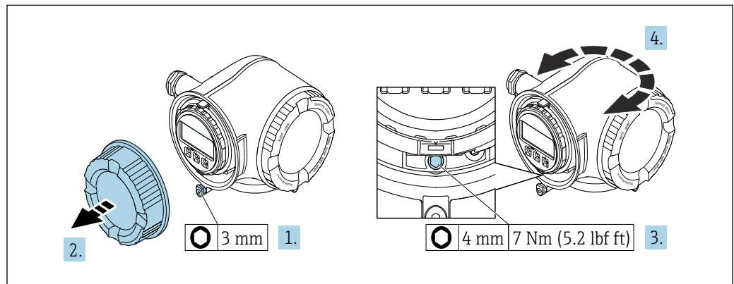
図 10 非防爆ハウジング
