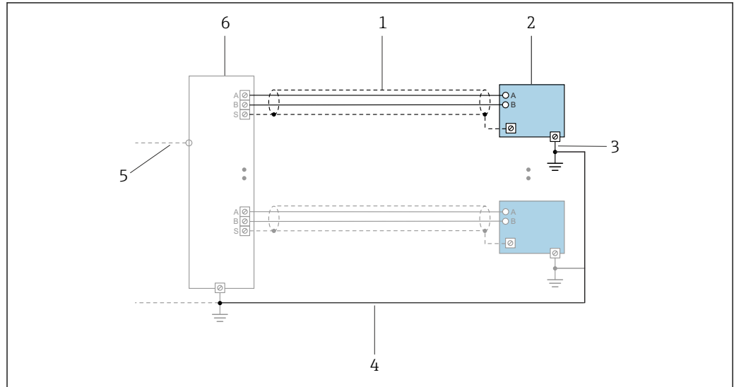
図 13 PROFINET (Ethernet-APL 対応) の接続例
