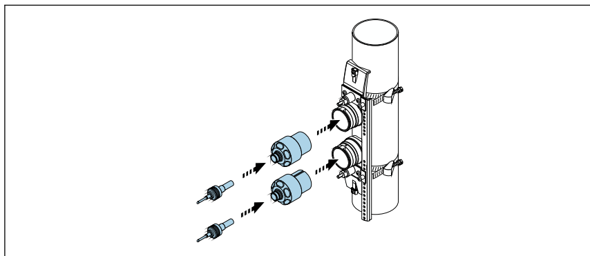
24 Монтаж датчиков и подключение кабелей датчика
