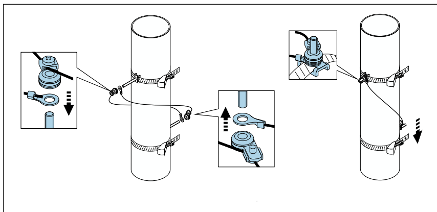
17 Размещение стяжных лент (этапы 2–4)
