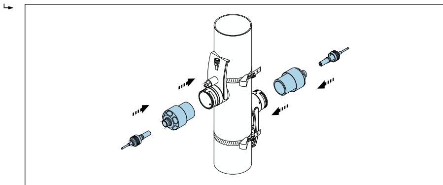
21 Монтаж датчиков и подключение кабелей датчика
