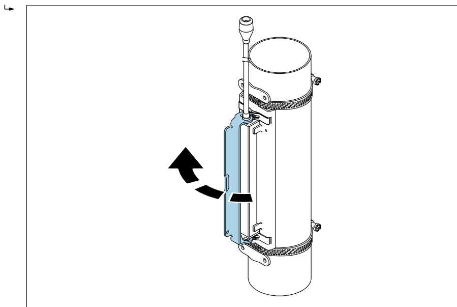
15 Закрепление корпуса датчика
