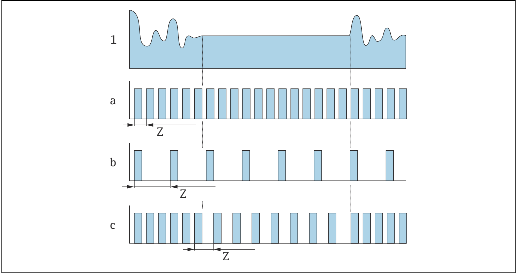
15 Arbeitsweisen der unterschiedlichen Messwerterfassungen
