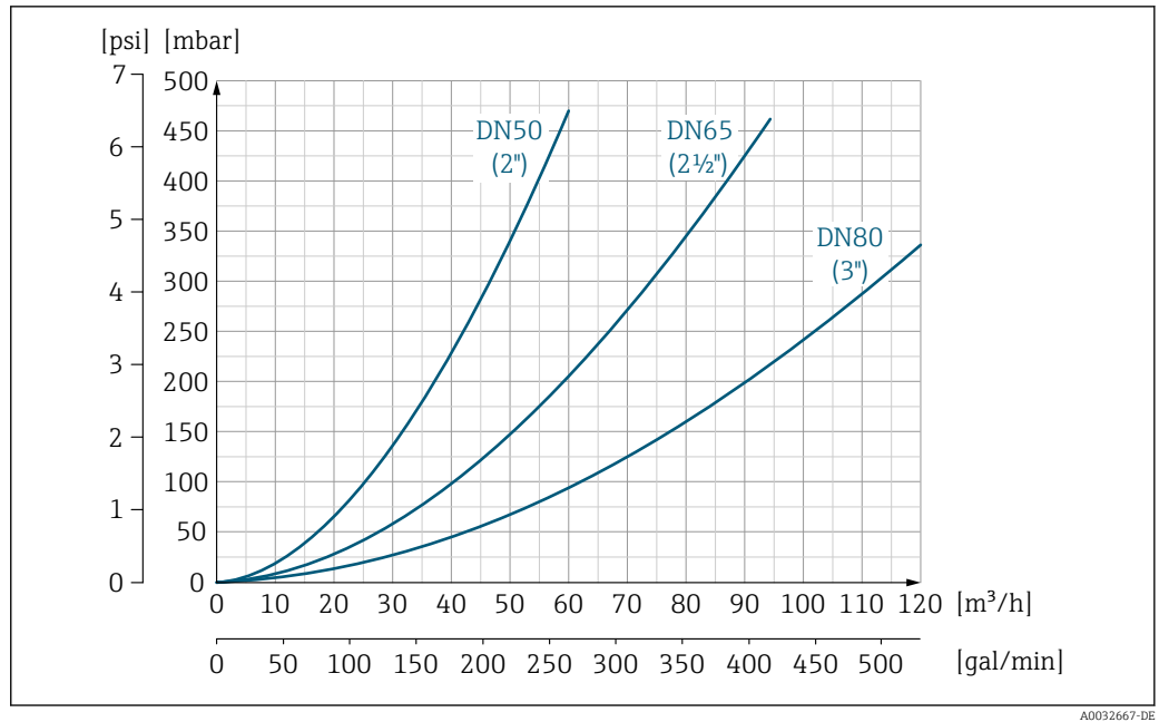
17 Druckverlust DN 50 ... 80 (2 ... 3") bei Bestellmerkmal "Bauart", Option C "Festflansch, Messrohr eingeschnürt, 0 x DN Ein-/Auslaufstrecken"
