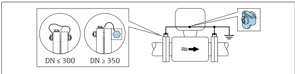
7 Potenzialausgleich über Erdungsklemme und Rohrleitungsflansche
