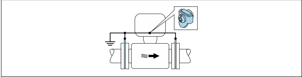
図 5 接地端子およびアースリングを介した電位平衡 ( PE = P_{FL} = P_M )
