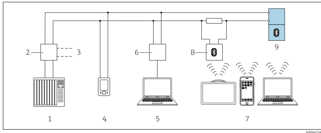
5 Möglichkeiten der Fernbedienung via HART-Protokoll
