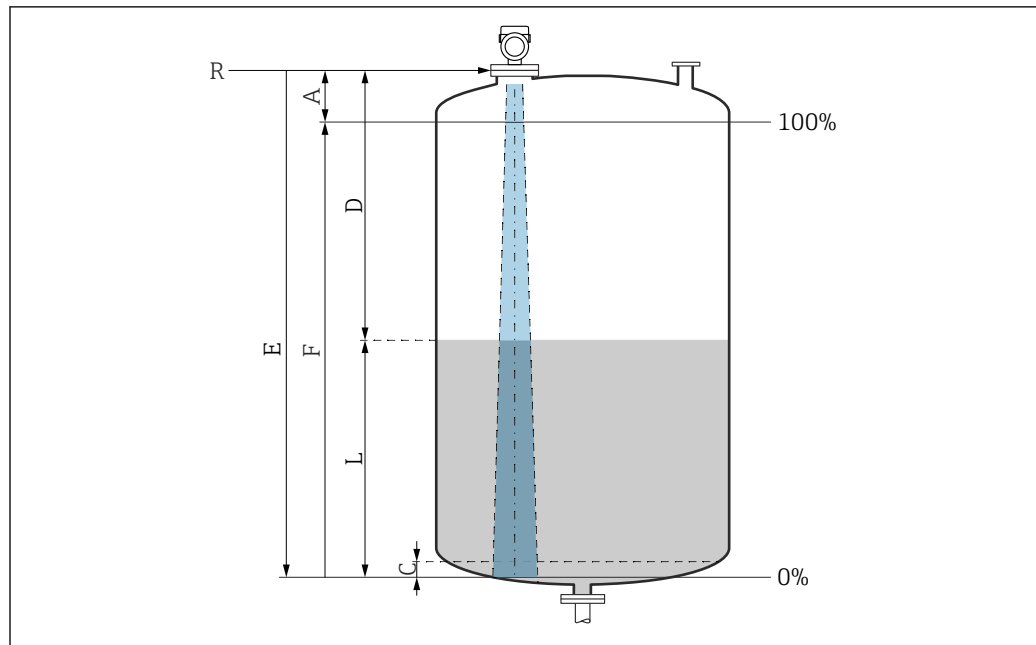
6 Konfigurationsparameter zur Füllstandmessung in Flüssigkeiten
