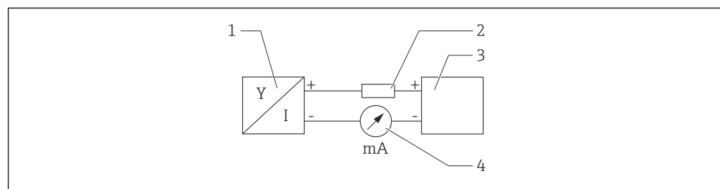
3 Blockschaltbild HART Anschluss
