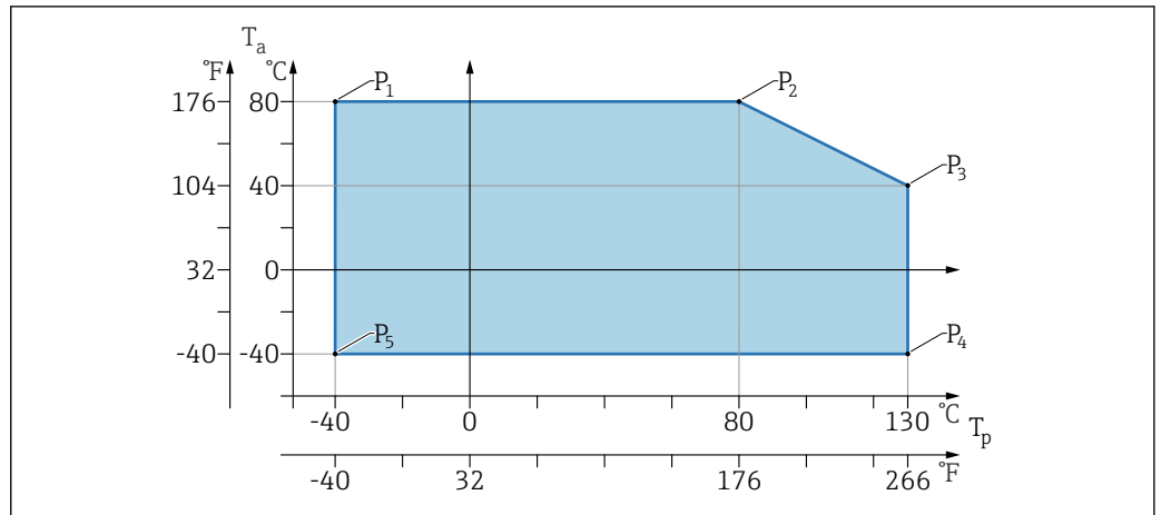
9 Umgebungstemperatur T_a in Abhängigkeit von der Prozessstemperatur T_p
