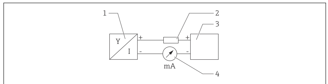
图 3 HART 信号回路接线图
