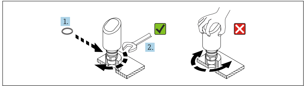
图 2 旋转拧入设备
