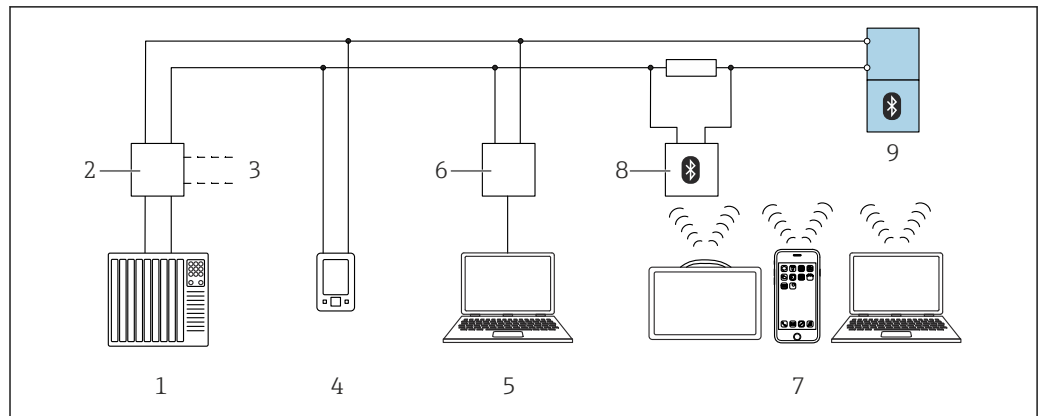
图 5 通过 HART 通信进行远程操作
