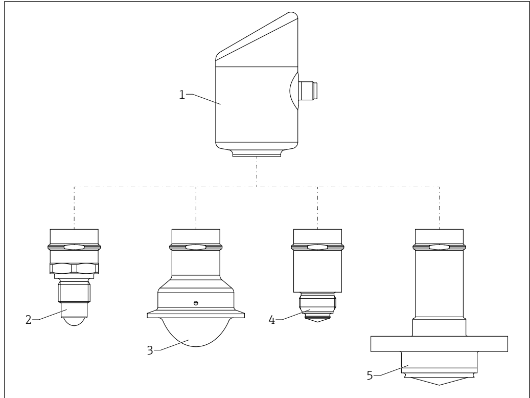
1 Diseño de producto Micropilot FMR43 con conexiones a proceso de muestra
