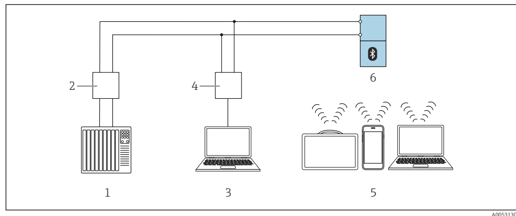
4 Opciones de funcionamiento remoto a través de IO-Link
