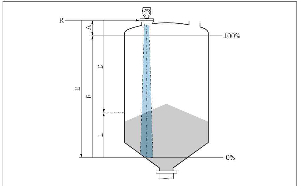
Fig. 6 Parámetros de configuración para la medición de nivel en sólidos granulados
