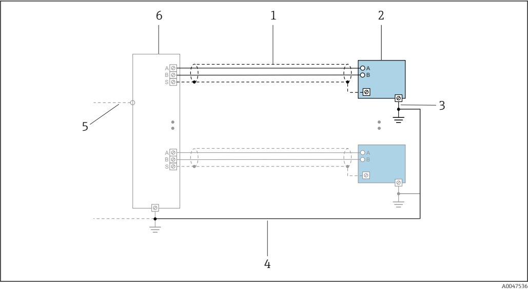
13 Ejemplo de conexión para PROFINET con Ethernet APL
