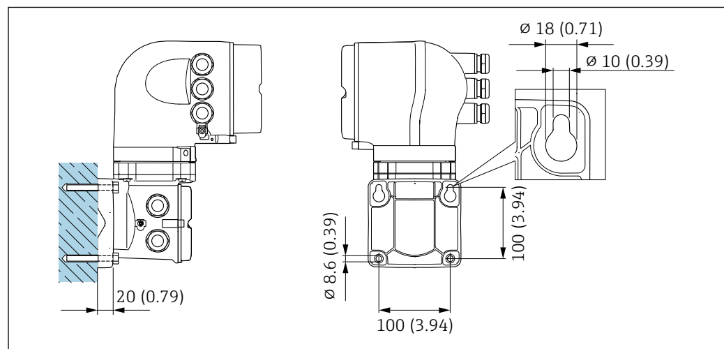
Fig. 13 Unità ingegneristica, mm (in)
