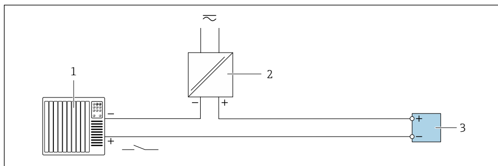
26 Esempio di connessione per ingresso di stato
