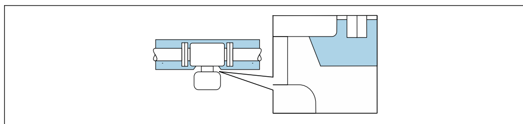
7 Coibentazione con collo di estensione non coibentato
