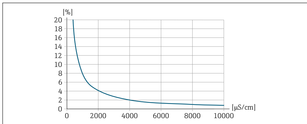
30 Wiederholbarkeit in % vom Messwert - Elektrische Leitfähigkeit [µS/cm]
