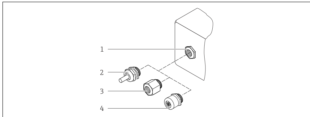
31 Mögliche Kabeleinführungen/-verschraubungen
