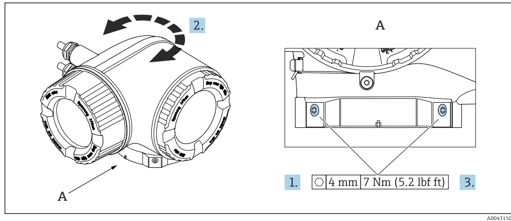
15 Boîtier Ex
