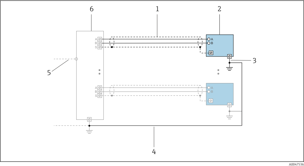
8 Ejemplo de conexión para PROFNET con Ethernet APL
