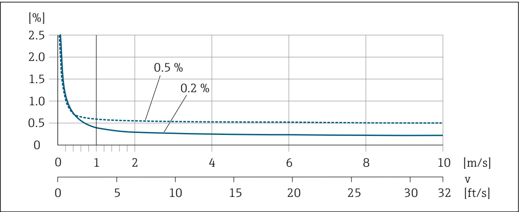
29 Error medido máximo en % lect.
