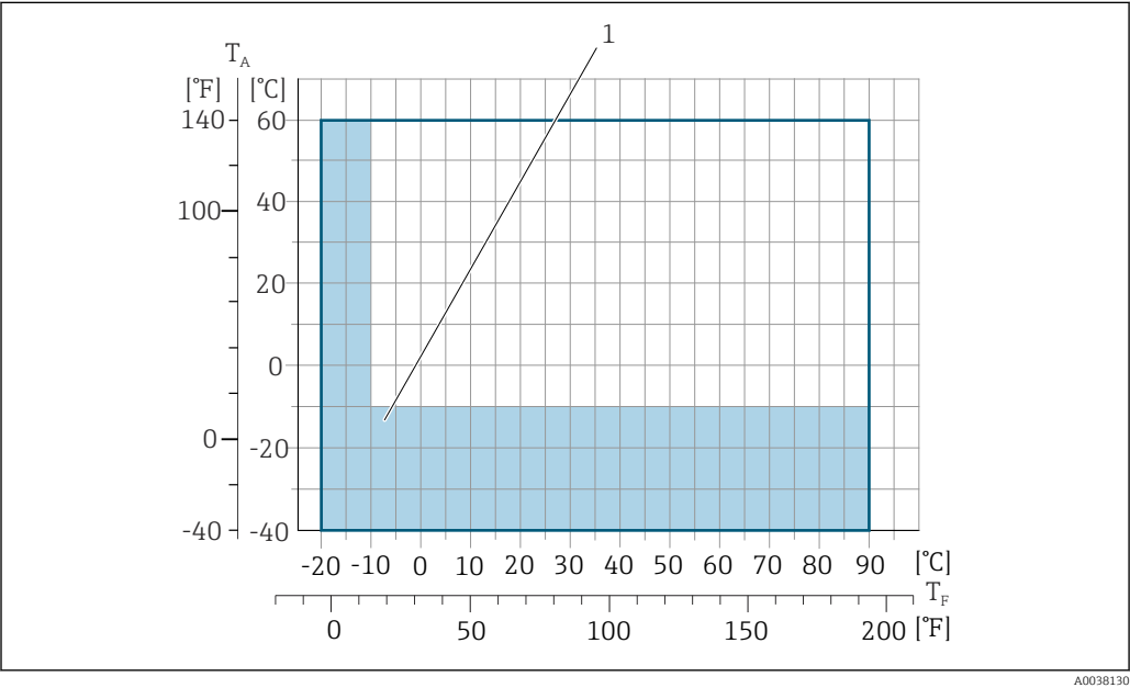
TA Temperatura ambiente TF Temperatura del producto 1 Área coloreada: El rango de temperatura ambiente de -10 ... -40 °C (+14 ... -40 °F) y el rango de temperatura del producto de -10 ... -20 °C (+14 ... -4 °F) son aplicables únicamente a las bridas inoxidables
