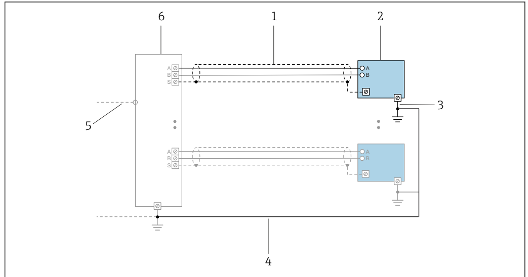
8 Ejemplo de conexión para PROFINET con Ethernet APL
