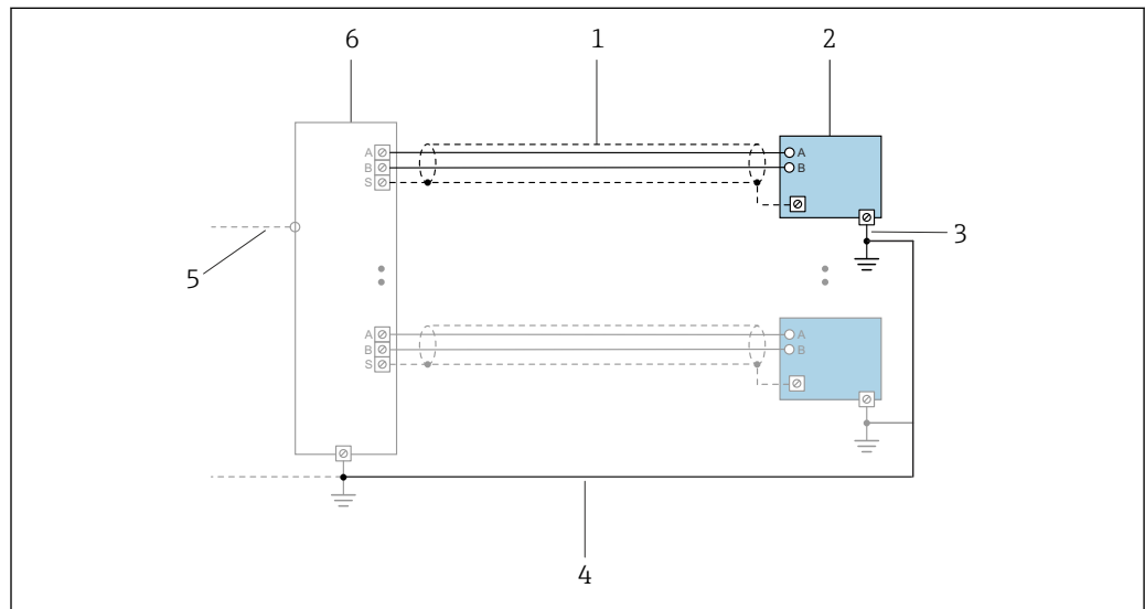
Fig. 15 Exemplo de conexão para PROFINET com Ethernet-APL
