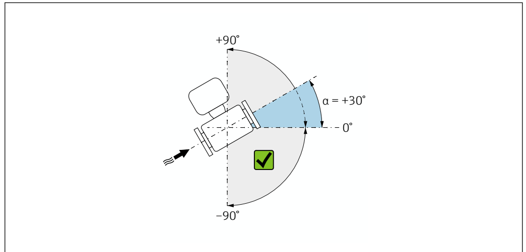
7 侧视图（介质流向为从左至右）
