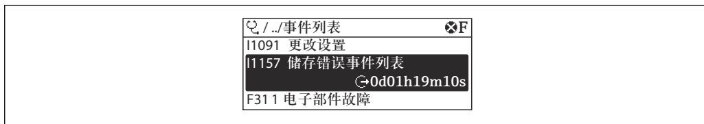
图 34 现场显示单元示例
