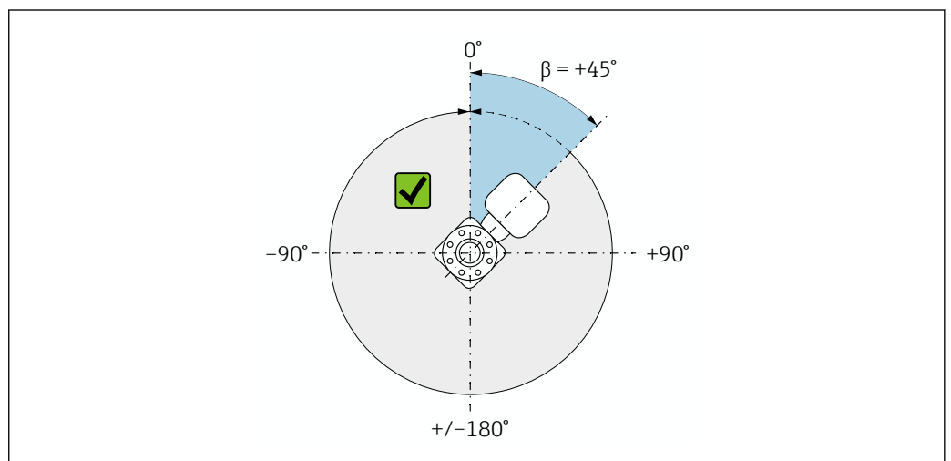
8 俯视图（顺着介质流向自上而下投影所得视图）
