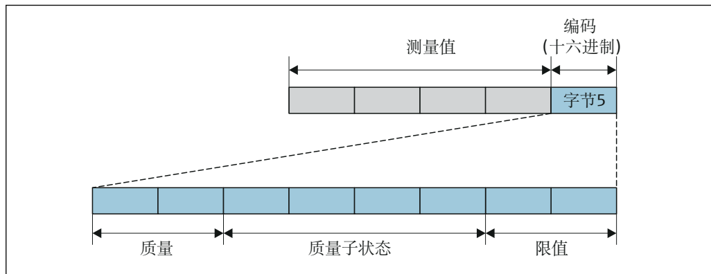
图 40 状态字节结构
