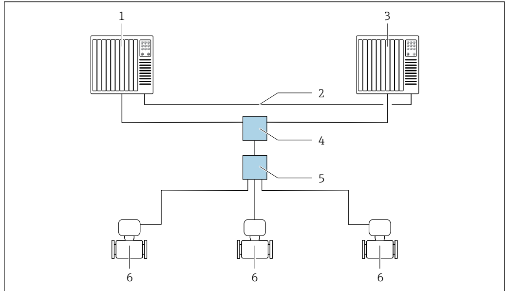
图 35 S2 系统冗余布局实例：星形拓扑结构
