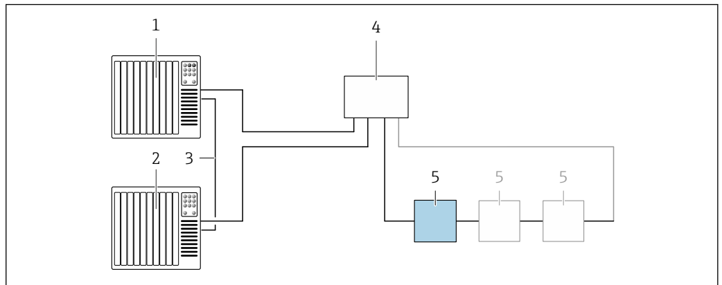
图 19 S2 系统冗余的连接示例
