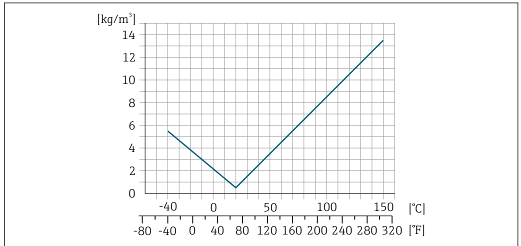
图 43 现场密度校正，例如在+20 °C (+68 °F)时
