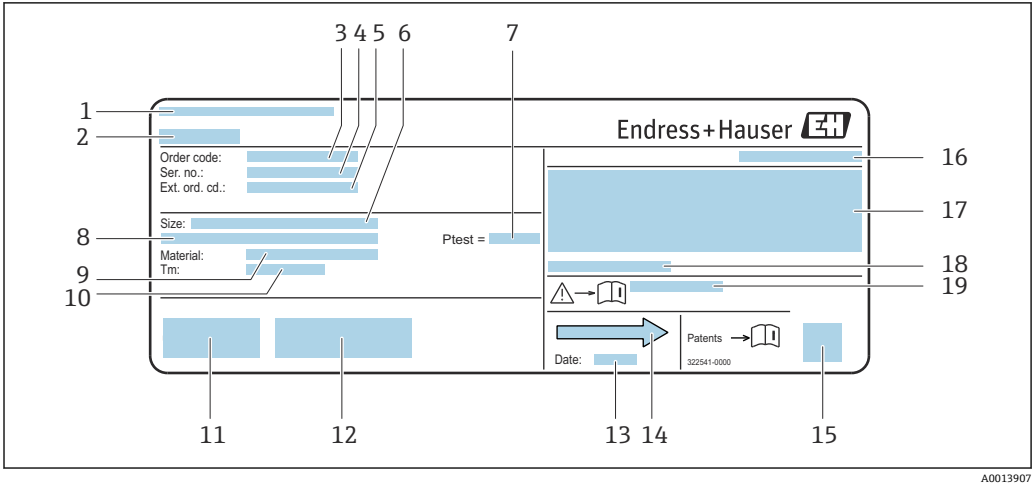
图 5 传感器的铭牌示意图
