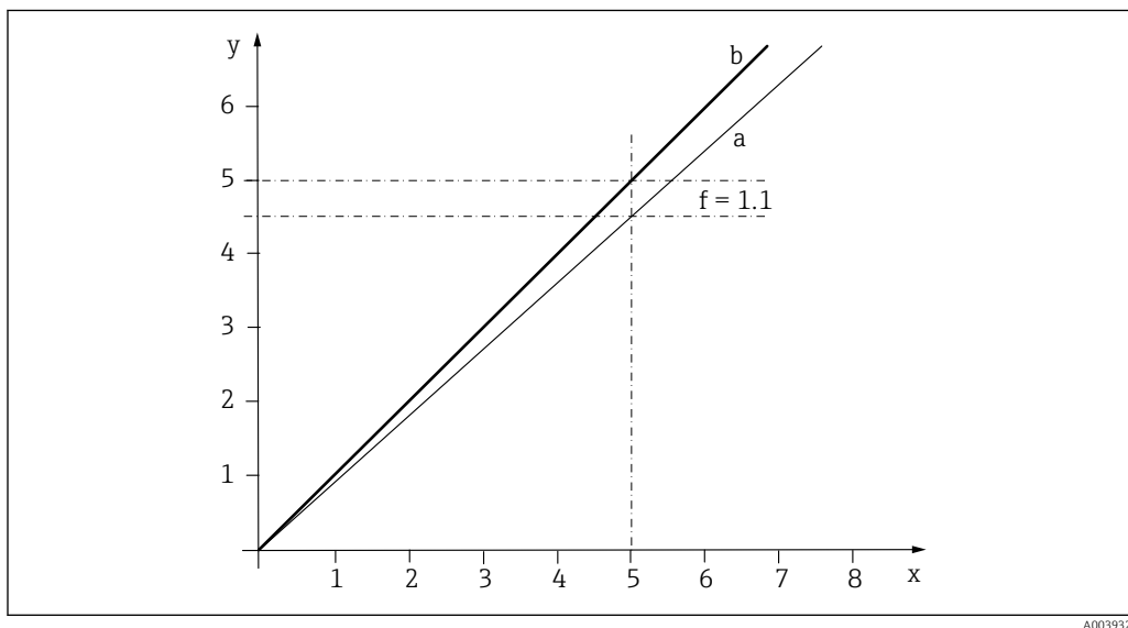
27 Принцип калибровки с коэффициентом
