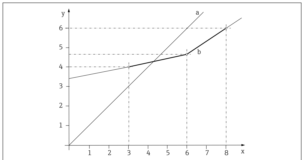
26 Принцип многоточечной калибровки (3 точки)
