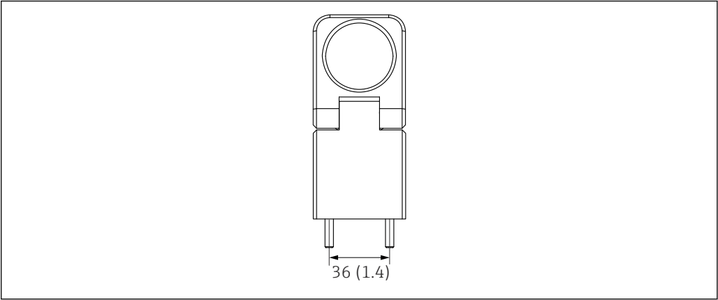
6 Размеры кольцевого зажима с проставкой. Единица измерения: мм (дюйм)
