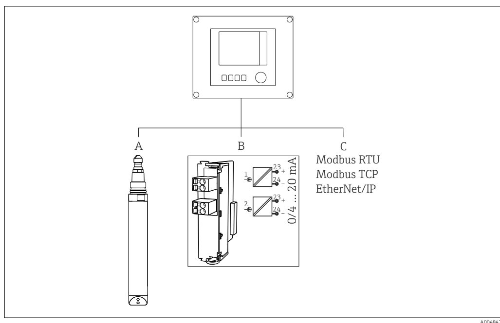
22 Варианты компенсации мутности
