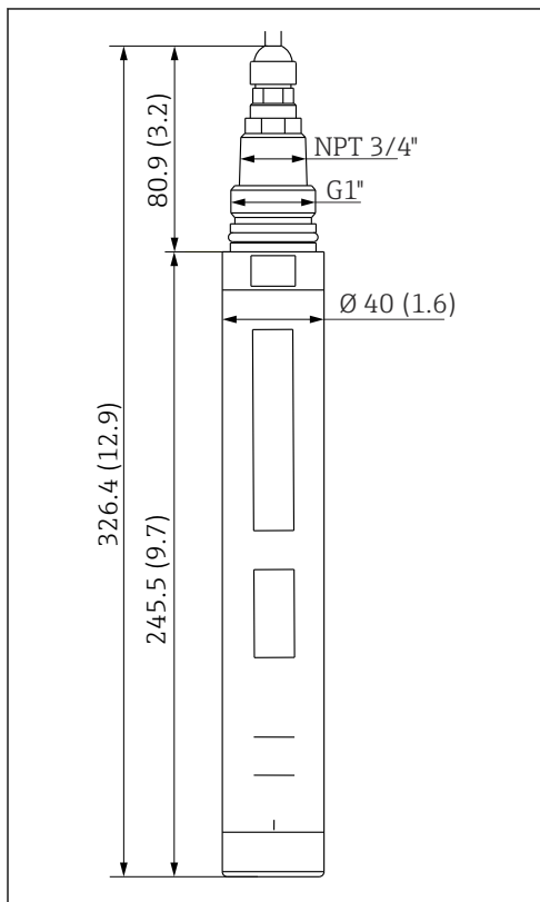
2 Размеры датчика. Единица измерения: мм (дюйм)
