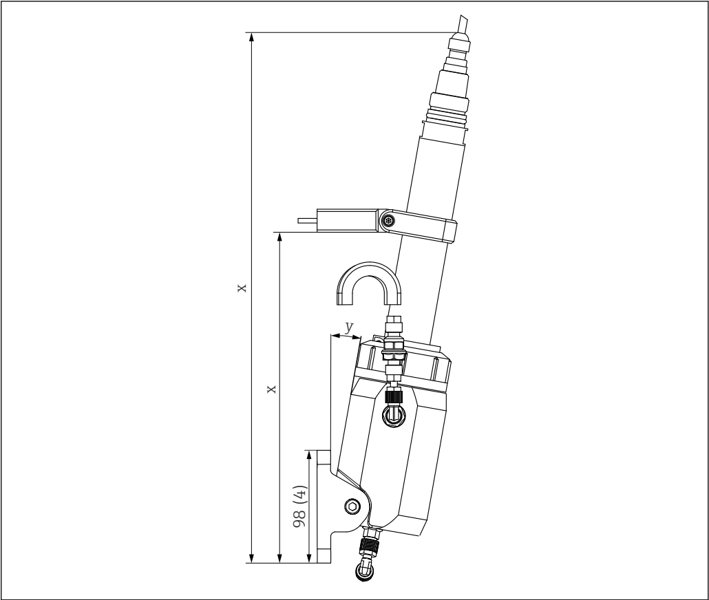
5 Размеры установленного датчика с арматурой. Единица измерения: мм (дюйм)
