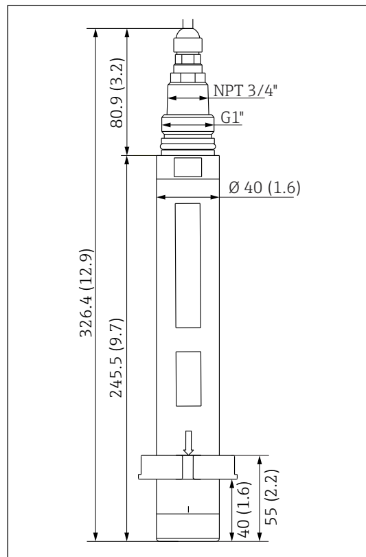
3 Размеры датчика с зажимным кольцом. Единица измерения: мм (дюйм)
