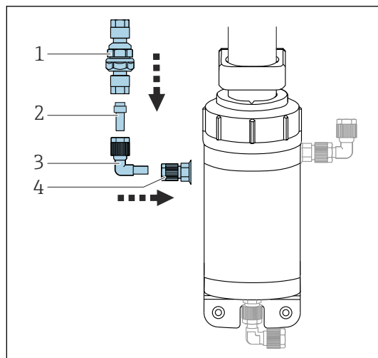
16 Установка очистного соединения
