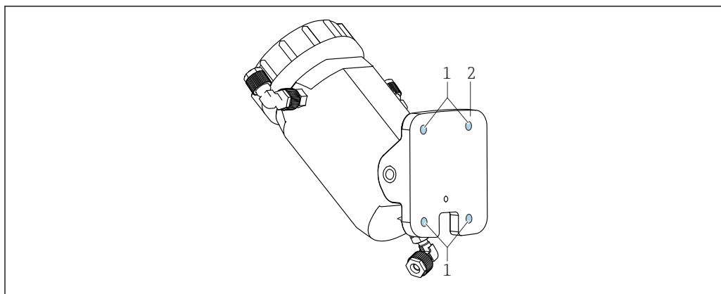
■ 14 Вид арматуры сзади
