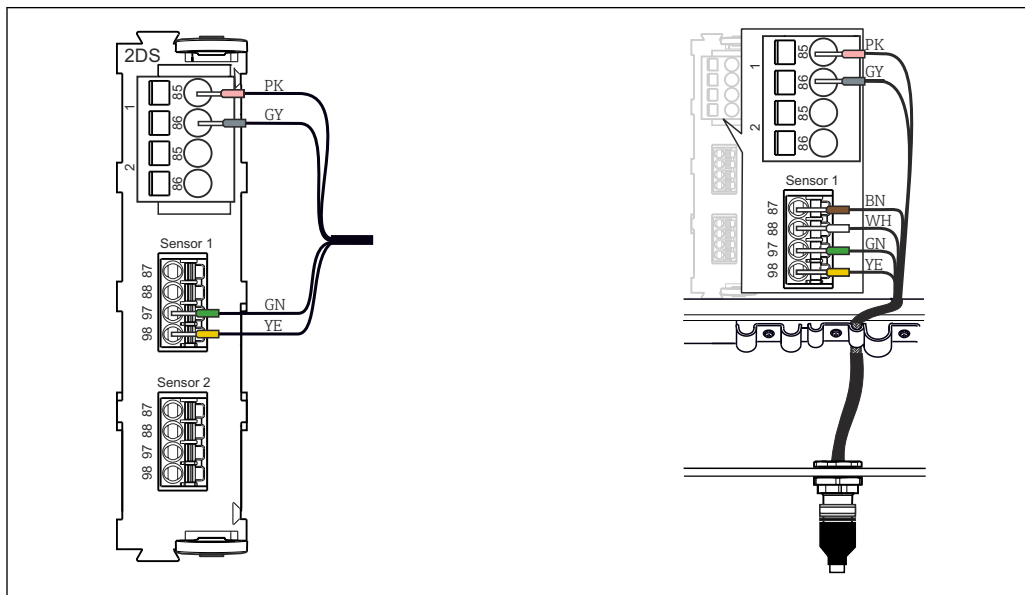
18 Подключение прибора к входу (слева) или с помощью разъема M12 (справа)
