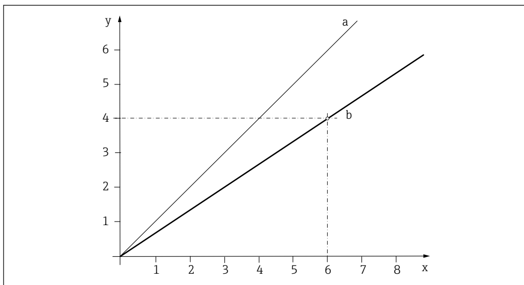
24 Принцип калибровки по 1 точке
