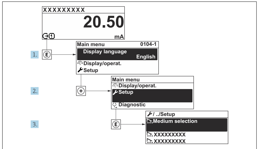
图 36 现场显示单元示例
