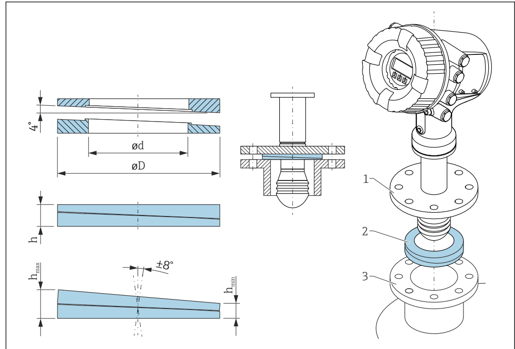
図 4 可変フランジシール (機器の角度を \pm 8^\circ 調節可能)
