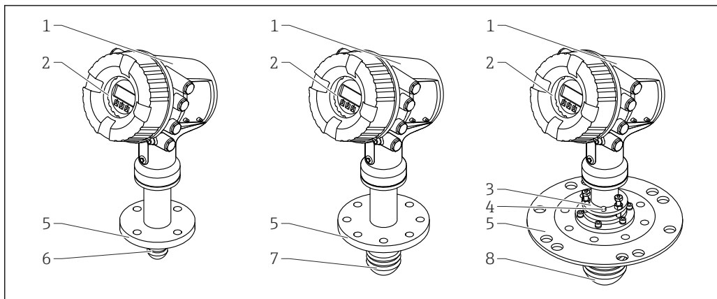
図 1 Micropilot NMR81 の構成
