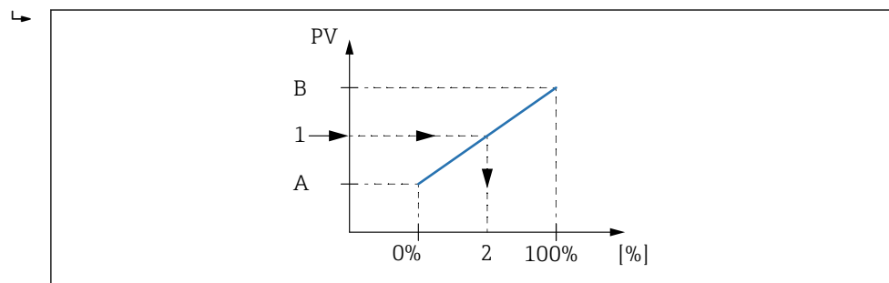
図 43 割合へのタンク変数のスケーリング
