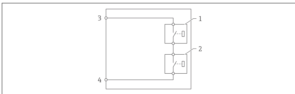
図 56 デジタル出力の 2 つのリレー
