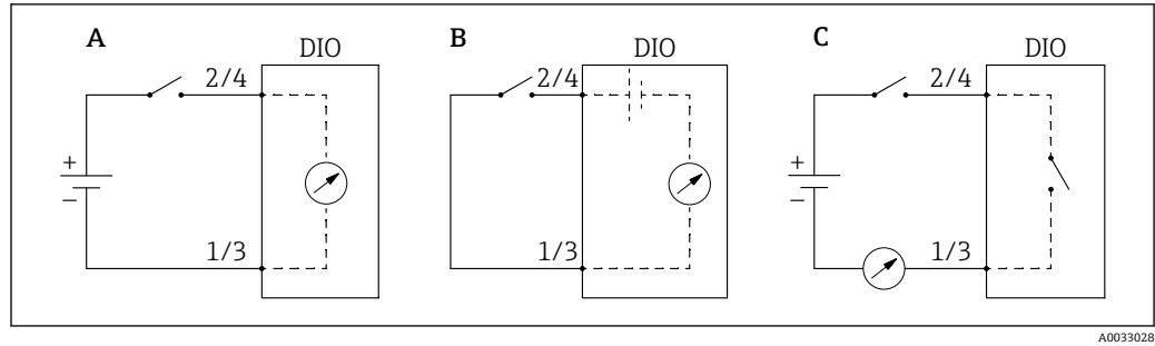
図 55 デジタル I/O モジュールの操作モード
