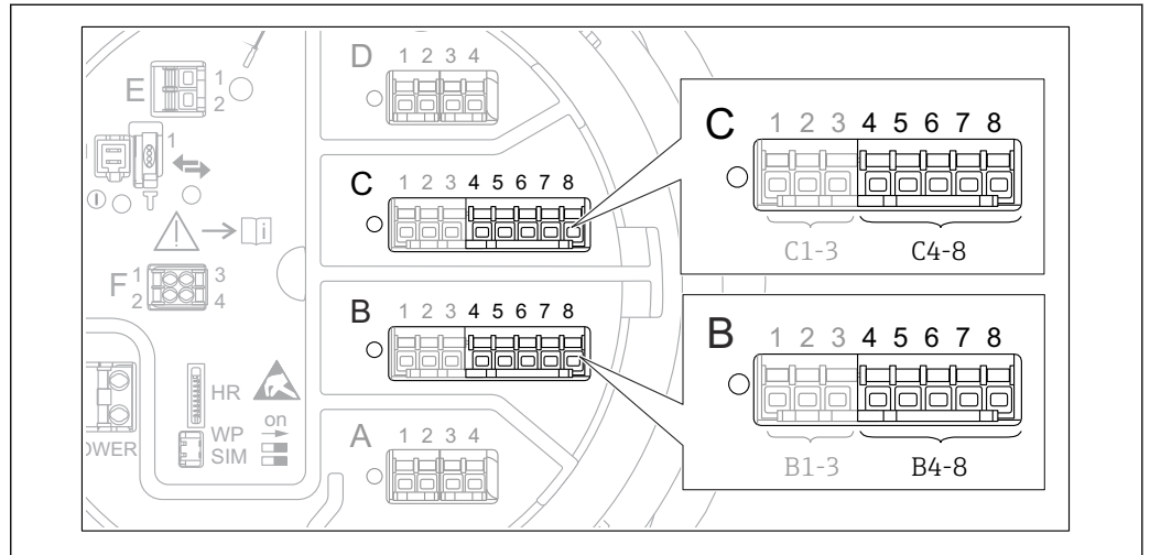
図 52 「Analog IP」 サブメニュー用端子 (それぞれ「B4-8」または「C4-8」)
