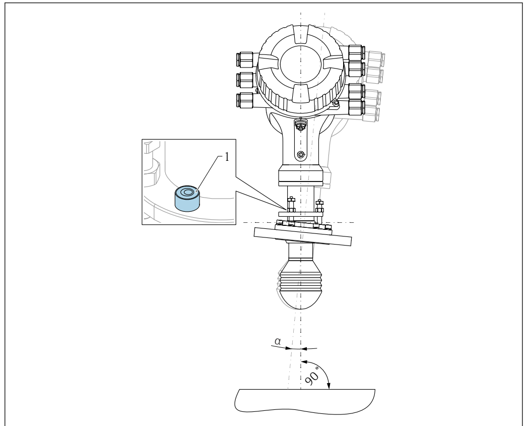
図 5 100 mm (4") アンテナの調節用ユニット
