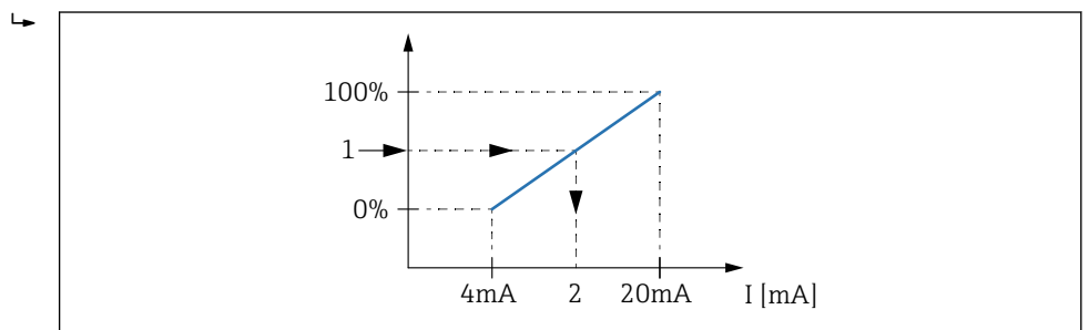
図 42 出力電流へのタンク変数のスケールリング
