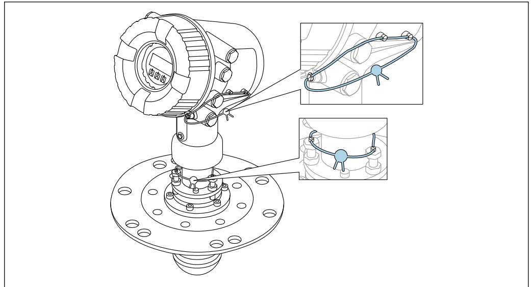
図 23 端子部（上部）および調節用ユニット（下部）のカバーのシーリング
