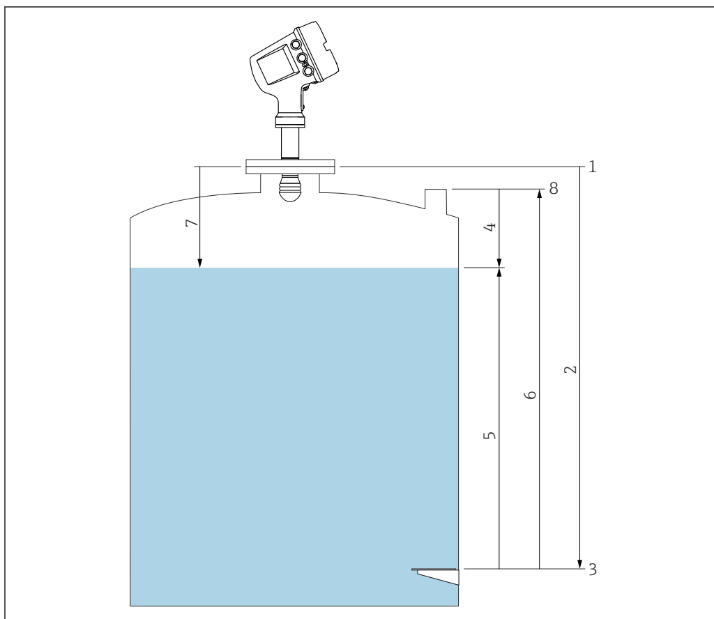
図 27 レーダータンク測定に関連する用語
