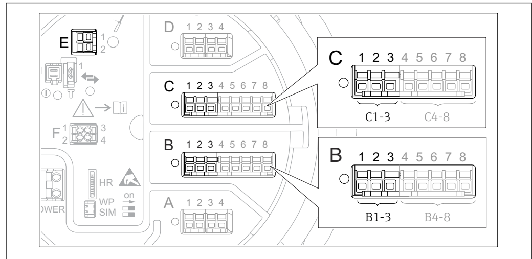
図 28 HART ループに使用可能な端子
