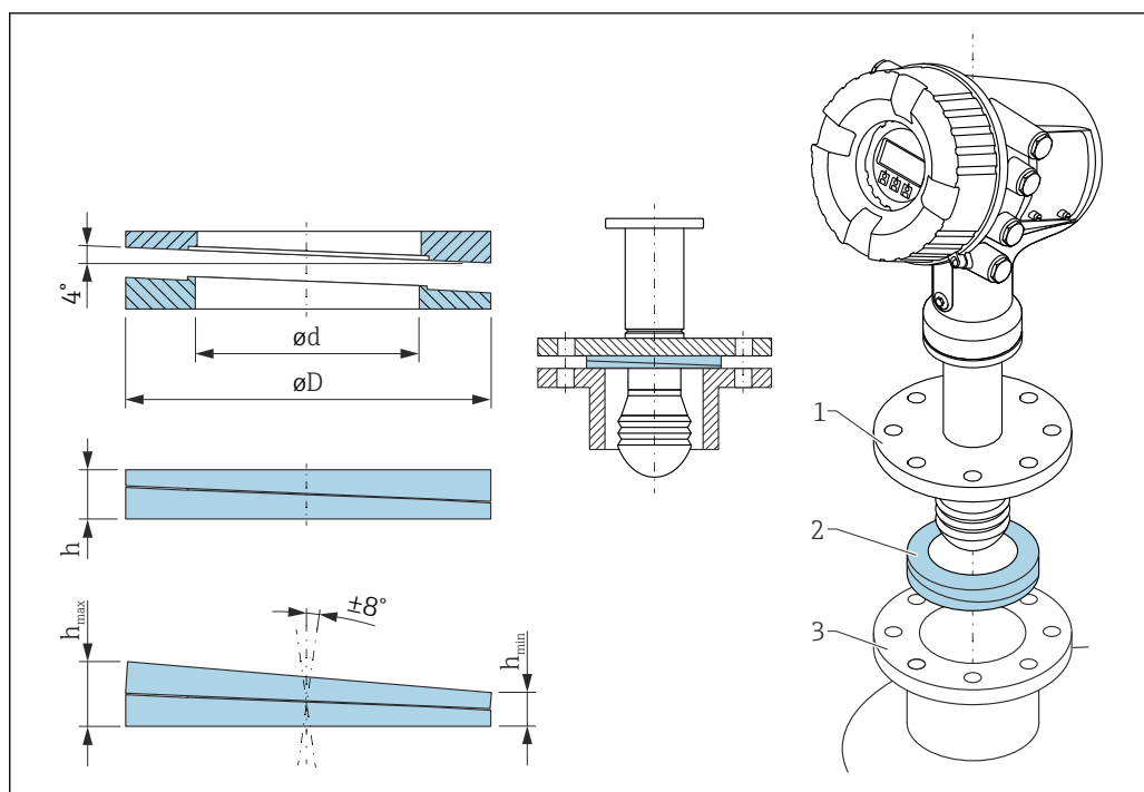
図 51 可変フランジシール（機器の角度を \pm 8^\circ 調節可能）
