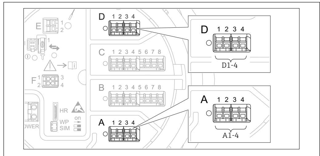
図 57 機器バージョンに応じて、「Modbus」、「V1」、「WM550」モジュール（例）がスロット B または C に対応する場合があります。
