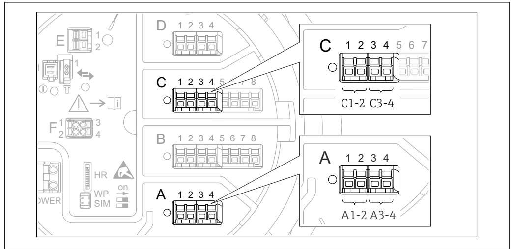
図 47 デジタル I/O モジュールの使用可能な端子 (例)。オーダーコードではデジタル I/O モジュールの数と端子を指定します → 図 24。
