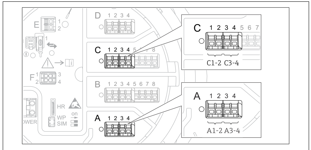
図 54 デジタル入力または出力の名称 (例)
