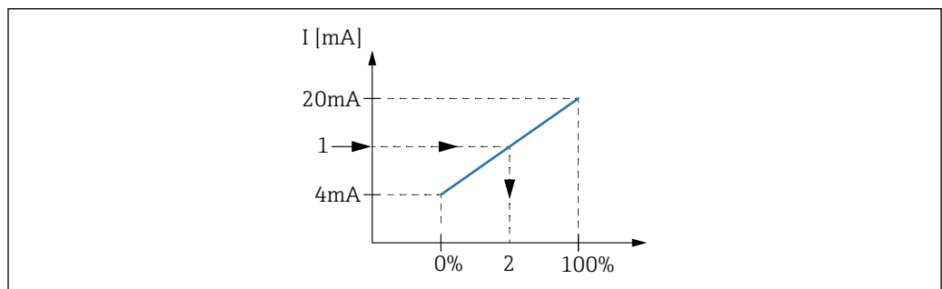
図 32 プロセス変数への 4~20 mA 入力のスケーリング
