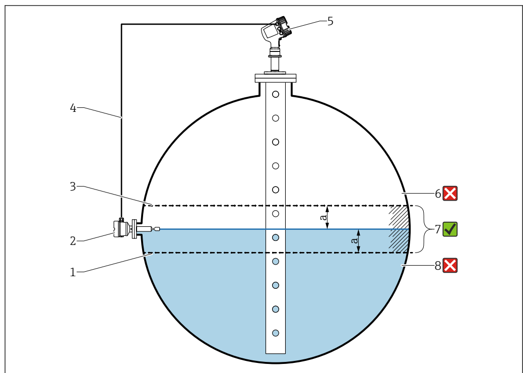
図 39 レベルスイッチを使用したアプリケーション事例
