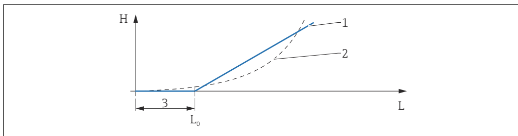
図 59 HyTD 補正の演算
