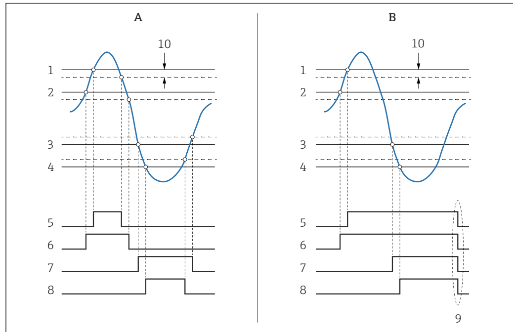
図 40 リミット評価の原理
