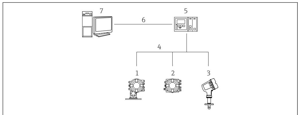
図 26 Tankvision Tank Scanner NXA820 経由でタンクゲージ機器を FieldCare に接続
