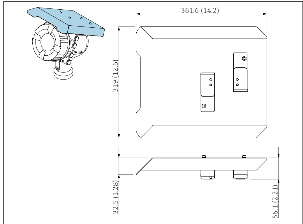
図 50 日除けカバー、寸法：mm (in)
