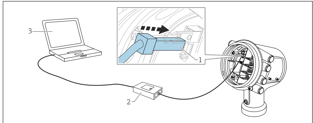
図 25 サービスインタフェース経由の操作
