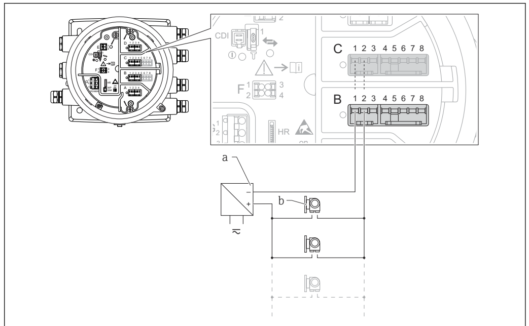
図 12 HART マスタモードのアナログ I/O モジュールのパッシブ使用
