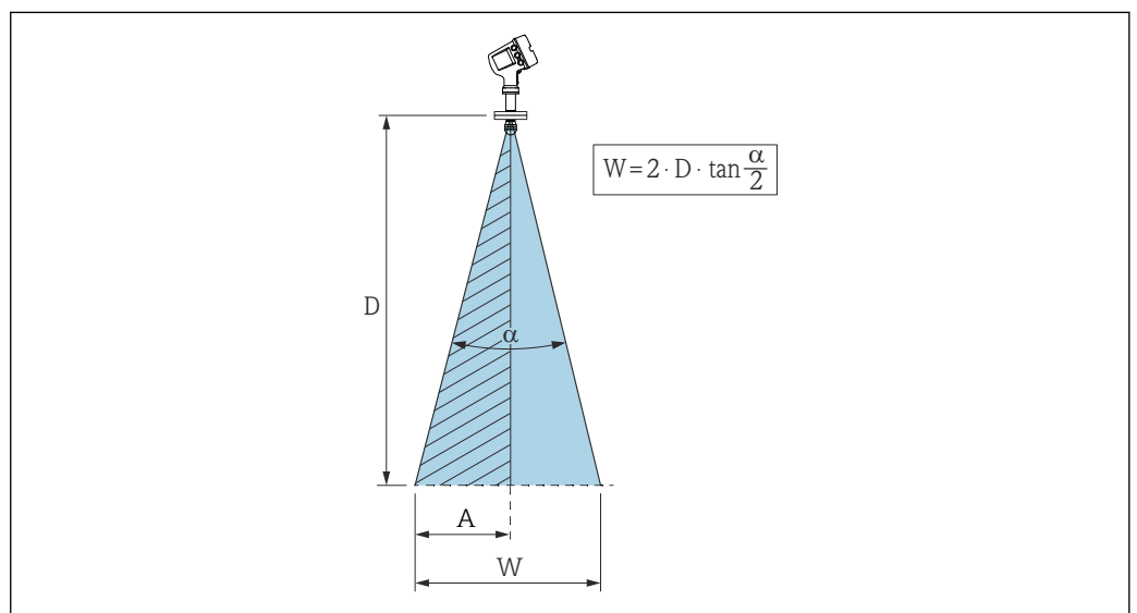
図3 放射角 \alpha 、距離 D およびビーム幅 W の関係。距離 A は、タンク内壁（または他の設置物）までの最小距離。距離 A は、ビーム幅 W の半分に等しい
