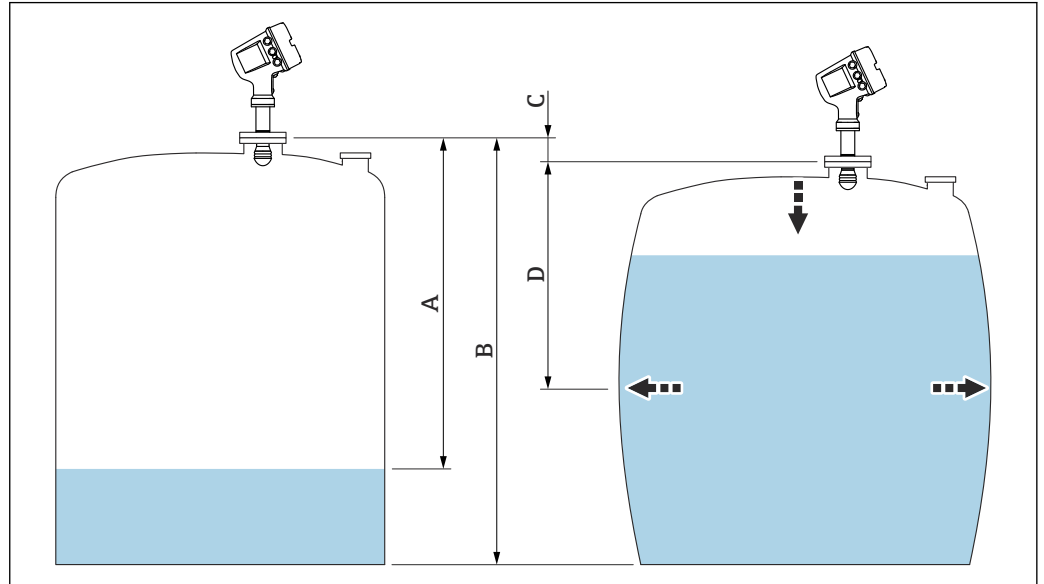
図 36 静圧タンク変形補正 (HyTD)
