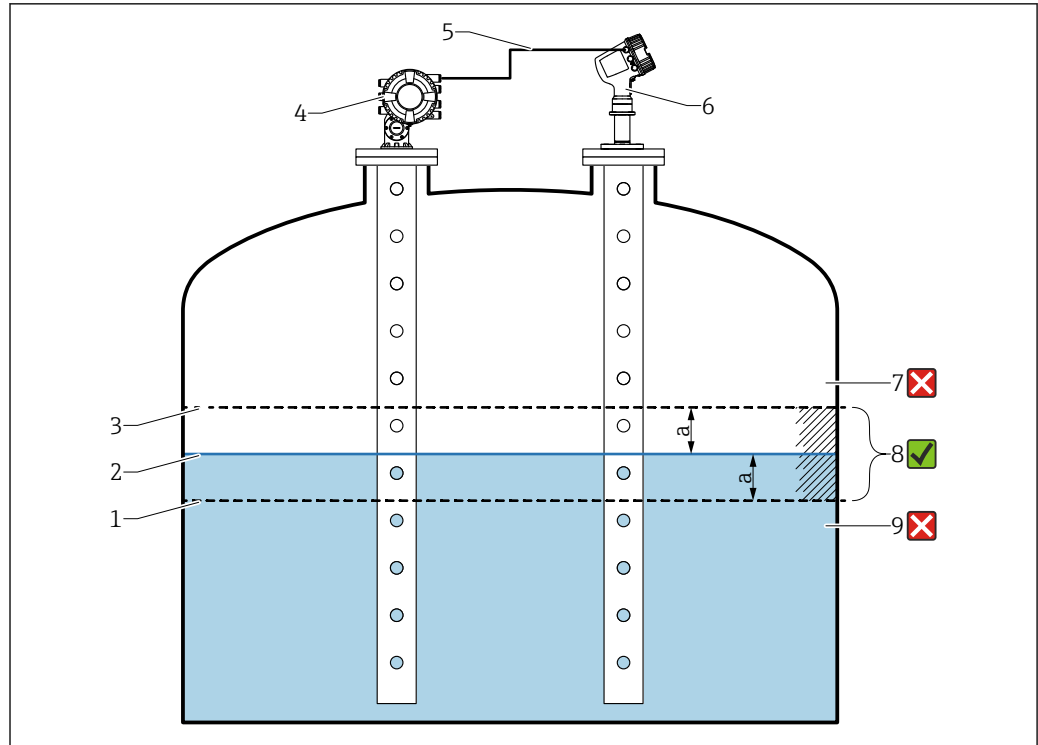
図 37 Proservo NMS8x を使用したアプリケーション事例
