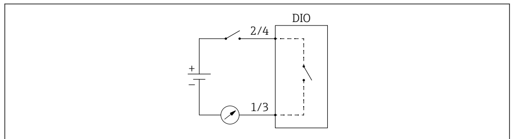
図 48 デジタル出力としてデジタル I/O モジュールの使用方法
