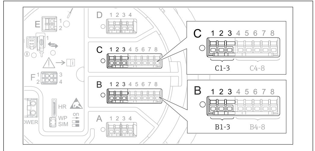
53 「Analog I/O」サブメニュー用端子 (それぞれ「B1-3」または「C1-3」)
