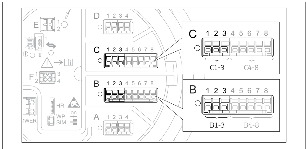
図 31 アナログ I/O モジュールの使用可能な端子。4~20 mA 入力として使用できます。機器のオーダーコードは、実際に存在するモジュールを示します → 図 24。
