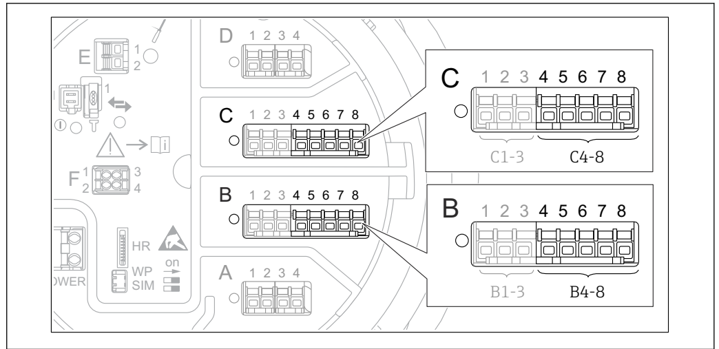
図 33 アナログ I/O モジュールの使用可能な端子。測温抵抗体を接続できます。機器のオーダーコードは、実際に存在するモジュールを示します → 図 24。
