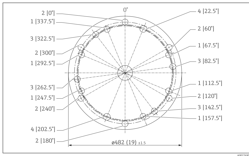
16 UNI-Flansch DN300/12"/300
