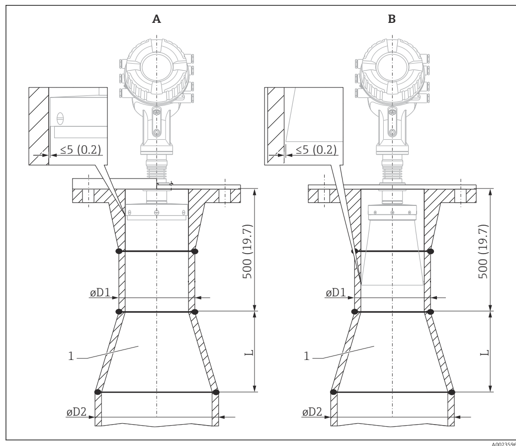
12 Installation des NMR84 in Schwallrohren mit größerem Durchmesser
