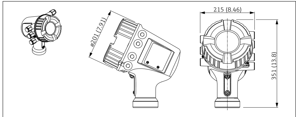
13 Abmessungen des Elektronikgehäuses; Maßeinheit: mm (in); Adapter für Kabeleinführungen sind in dieser Zeichnung nicht berücksichtigt.
