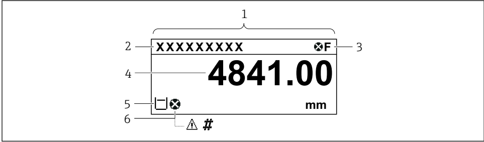
15 일반적인 기본 보기 모양(측정값 표시)
