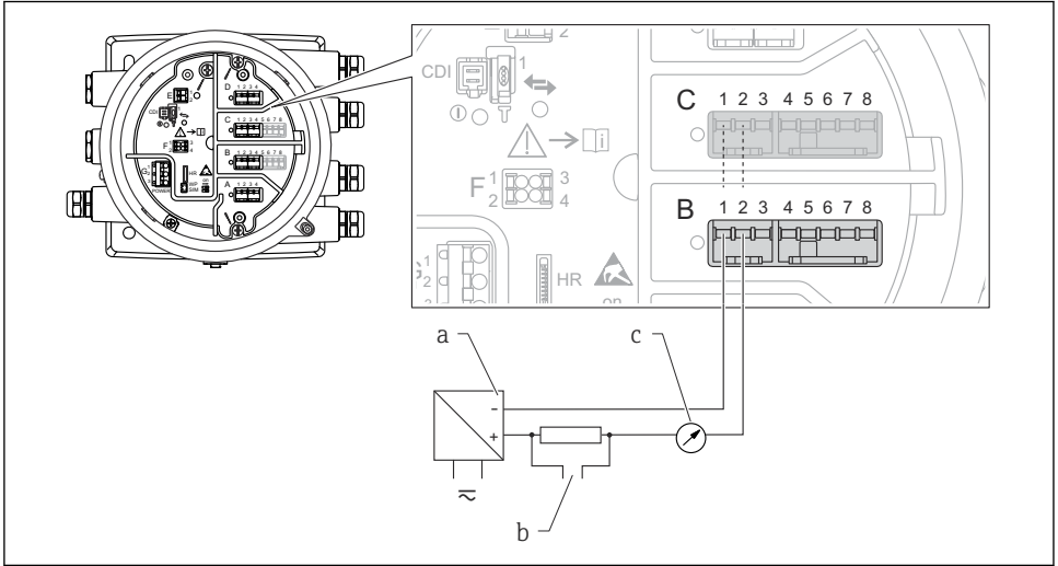
7 출력 모드에서 아날로그 I/O 모듈의 수동 사용
