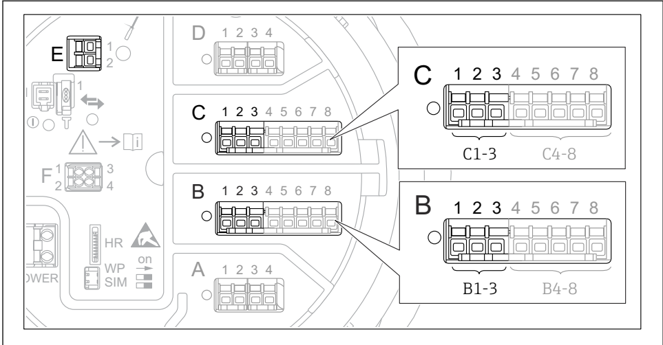
19 가능한 HART 루프 단자
