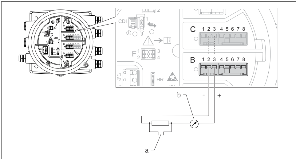
☐ 10 출력 모드에서 아날로그 I/O 모듈의 능동 사용
