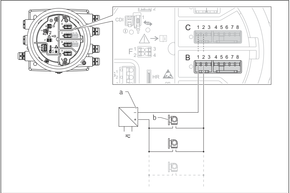
☐ 9 HART 마스터 모드에서 아날로그 I/O 모듈의 수동 사용
