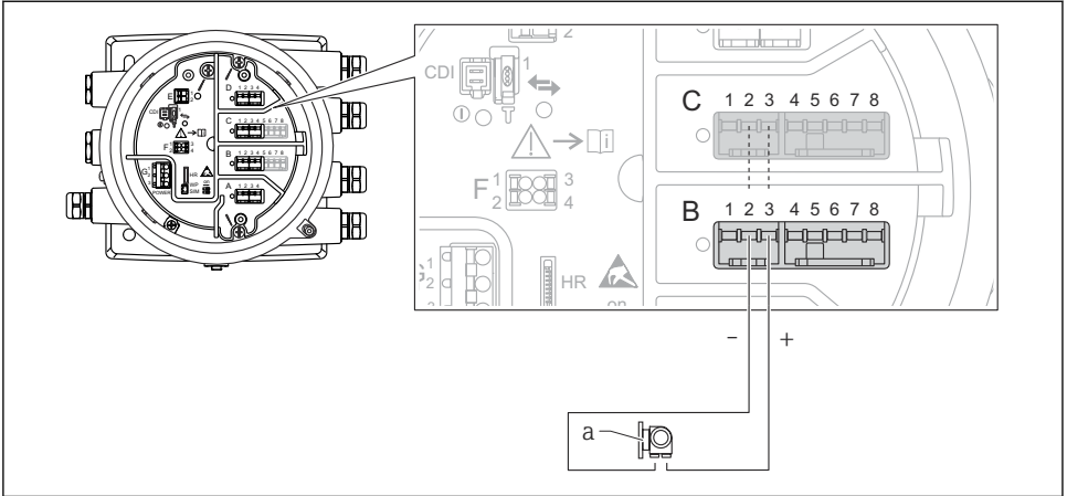
☐ 11 입력 모드에서 아날로그 I/O 모듈의 능동 사용
