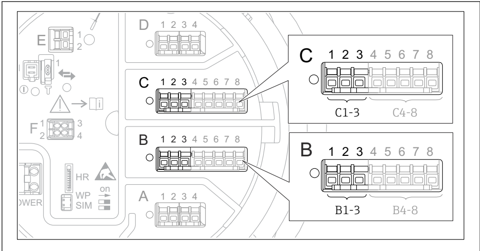
☞ 20 4-20mA 입력으로 사용할 수 있는 아날로그 I/O 모듈 위치. 계기 주문 코드에 따라 실제로 존재하는 모듈이 결정됩니다.
