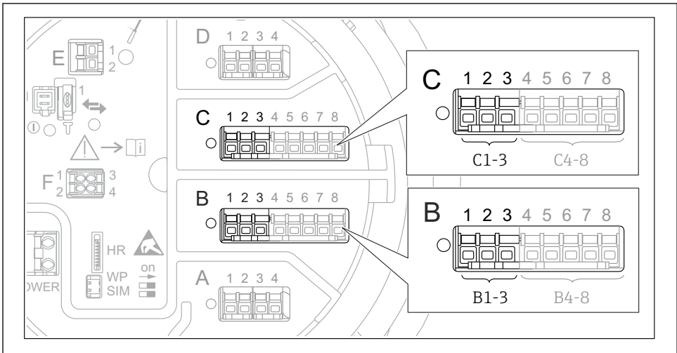
☞ 25 4~20 mA 출력으로 사용할 수 있는 아날로그 I/O 모듈 위치. 기기 주문 코드에 따라 실제로 존재하는 모듈이 결정됩니다.
