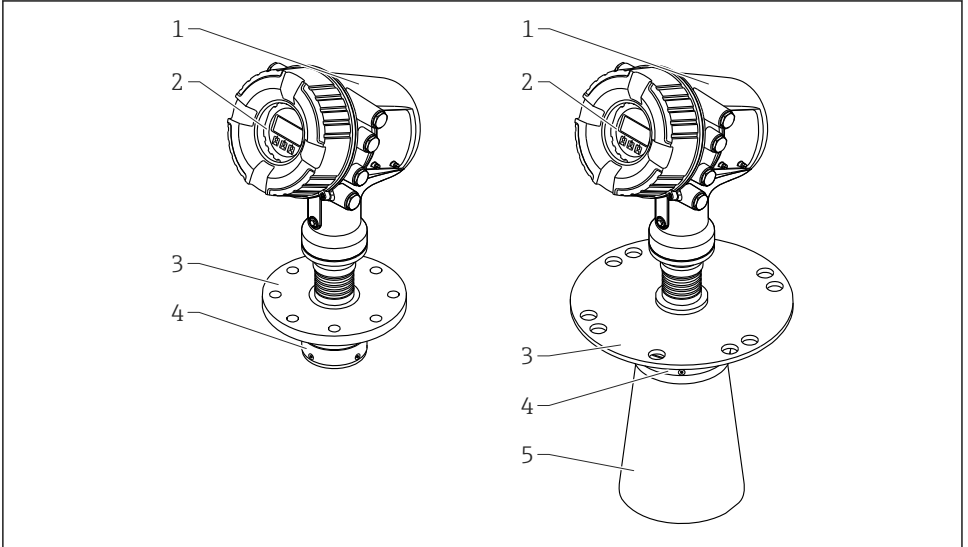
1 Micropilot NMR84의 디자인
