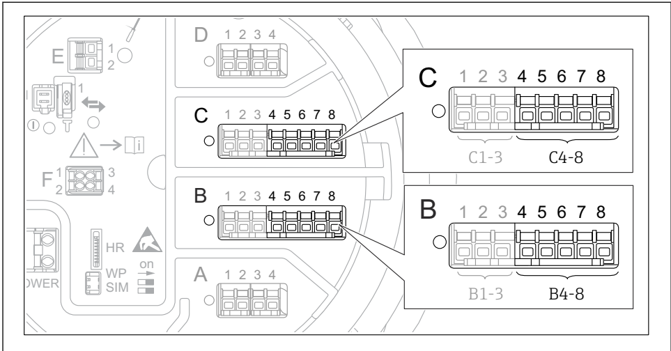
☞ 22 RTD를 연결할 수 있는 아날로그 I/O 모듈 위치. 계기 주문 코드에 따라 실제로 존재하는 모듈이 결정됩니다.
