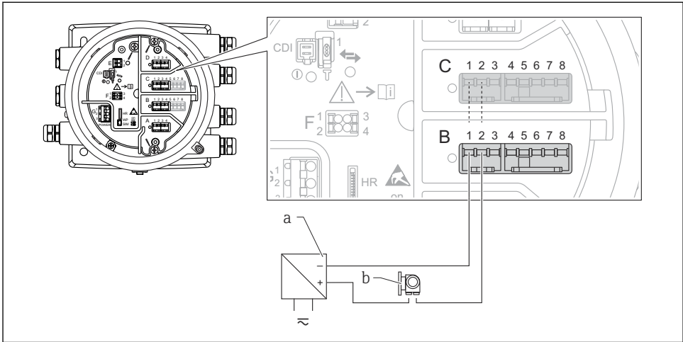
☞ 8 입력 모드에서 아날로그 I/O 모듈의 수동 사용
