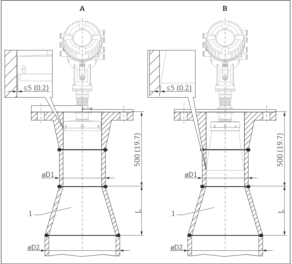
☐ 2 대직경 정수정에 NMR84 설치
