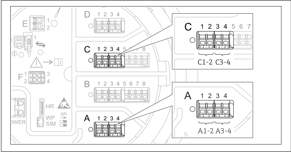
☞ 13 디지털 입력 또는 출력의 지정기호(예)
