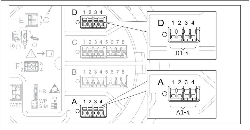
☐ 6 "Modbus", "V1" 또는 "WM550" 모듈의 지정기호(예); 계기 버전에 따라 이 모듈들을 슬롯 B 또는 C에도 끼울 수 있습니다.
