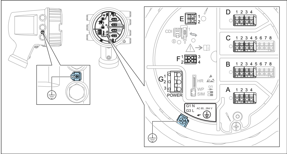
3 단자부(일반적인 예)와 접지 단자
