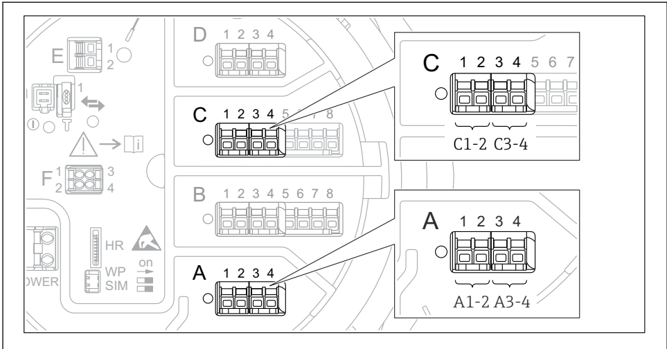
☐ 23 가능한 디지털 I/O 모듈 위치(예); 주문 코드에 따라 디지털 입력 모듈의 개수와 위치가 결정됩니다.
