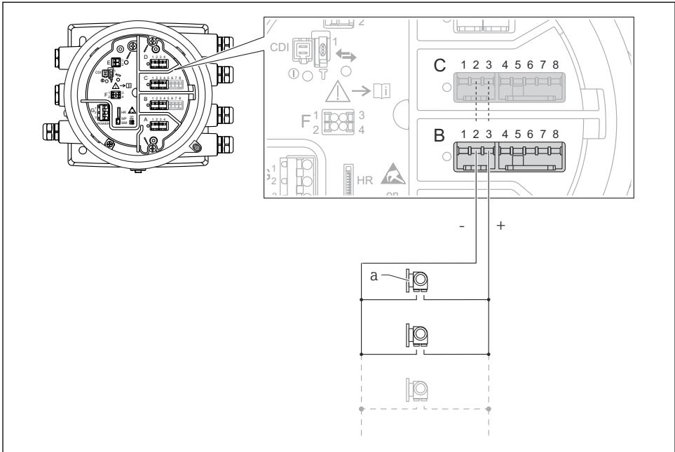
☐ 12 HART 마스터 모드에서 아날로그 I/O 모듈의 능동 사용
