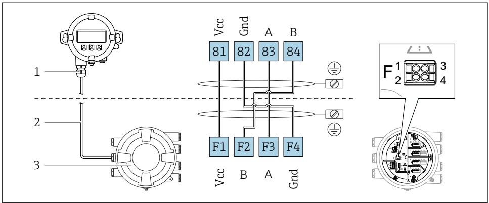
6 Conexão do display remoto e do módulo de operação DKX001 para o equipamento de tancaagem (NMR8x, NMS8x ou NRF8x)
