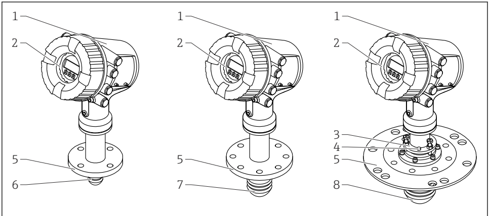
1 Desenho do Micropilot NMR81
