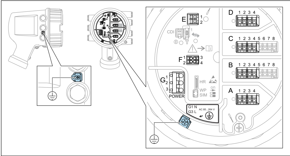
4 Compartimento do terminal (exemplo típico) e terminais de terra
