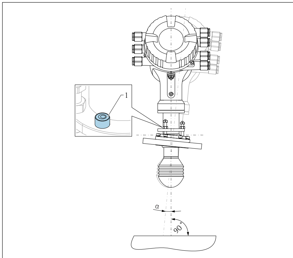
3 Dispositif d'orientation de l'antenne 100 mm (4")
