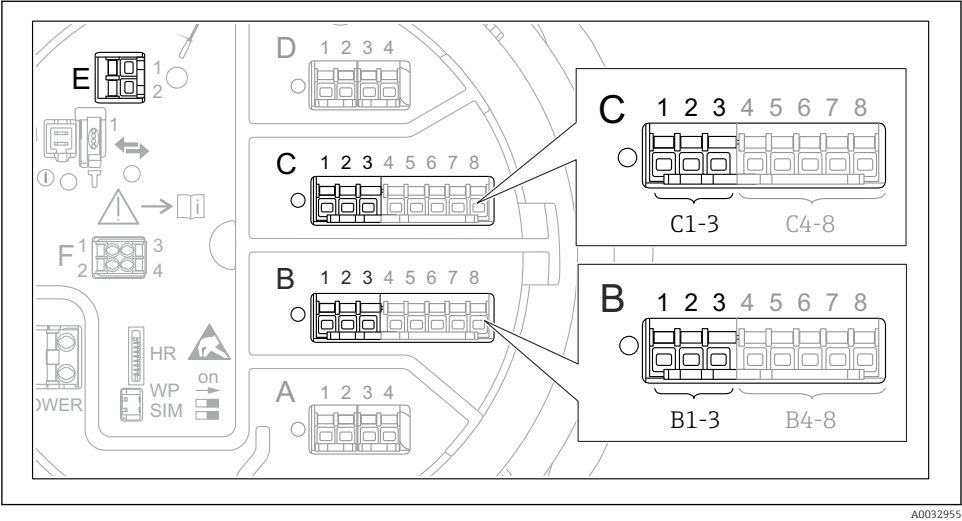
20 Bornes possibles pour les boucles HART
