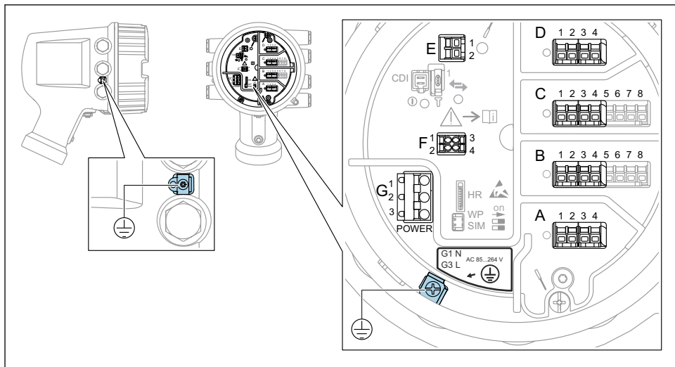
4 Compartiment de raccordement (exemple typique) et bornes de terre
