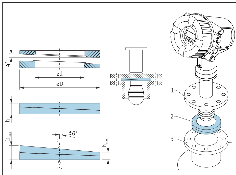
2 Joint réglable utilisé pour orienter l'appareil à \pm 8^\circ
