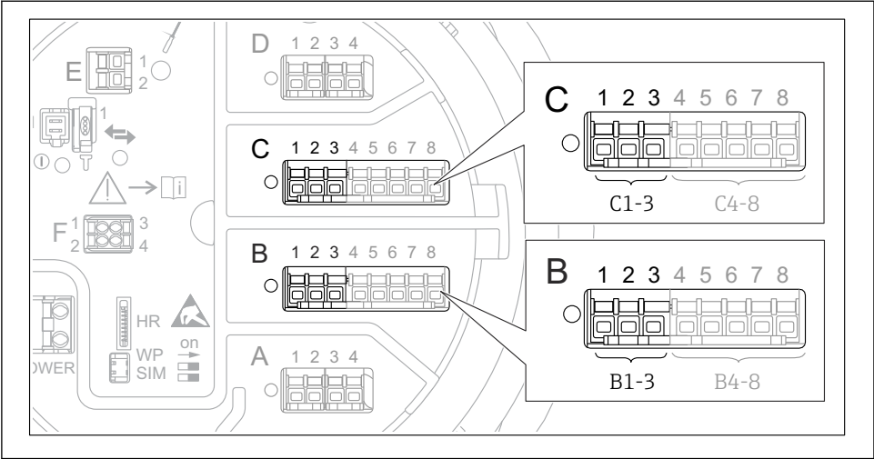
21 Emplacements possibles des modules Analog I/O, pouvant être utilisés comme entrée 4-20 mA. La référence de commande de l'appareil détermine le module réellement présent.
