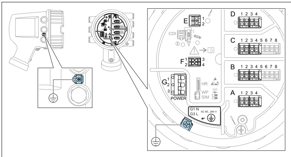
4 Клеммный отсек (типовой пример) и клеммы заземления
