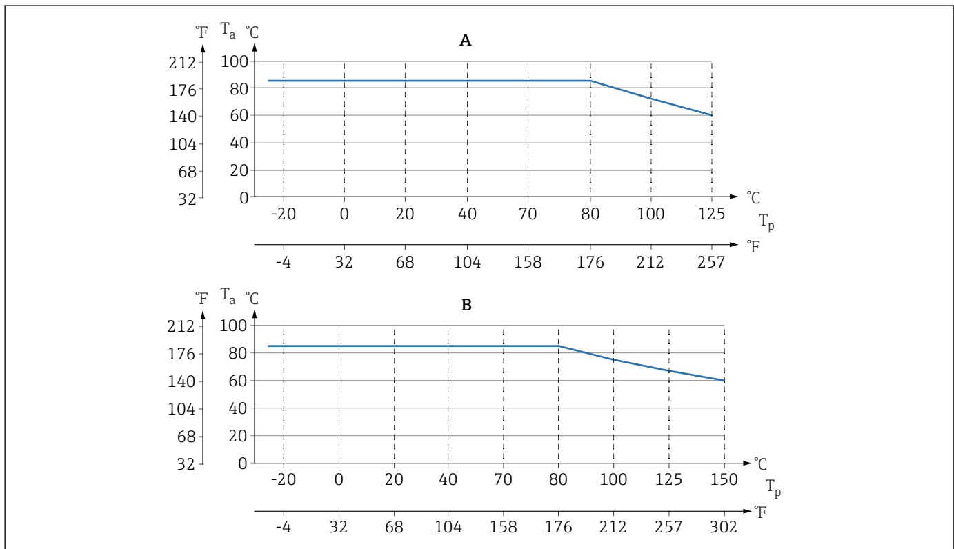
图 9 以上为无保温层垂直安装时的温度范围。
