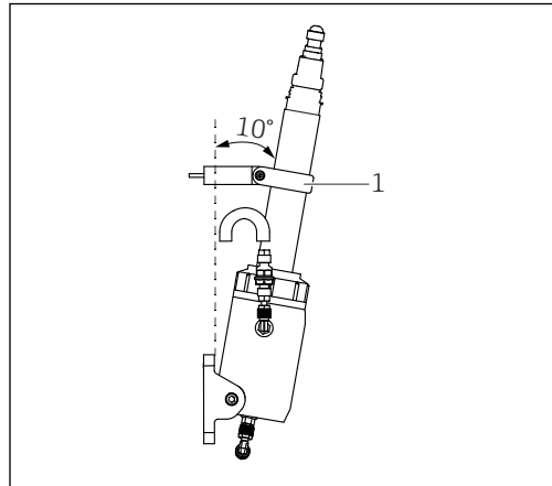
图 10 定位盘安装在上部，与安装板之间的相对角度为 10^\circ
