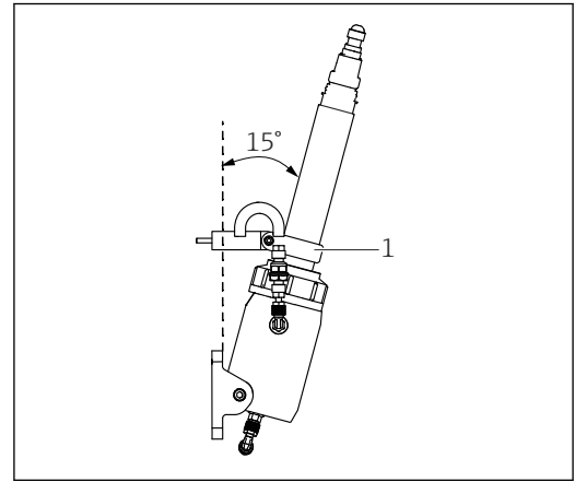
图 11 定位盘安装在下部，与安装板之间的相对角度为 15^\circ
