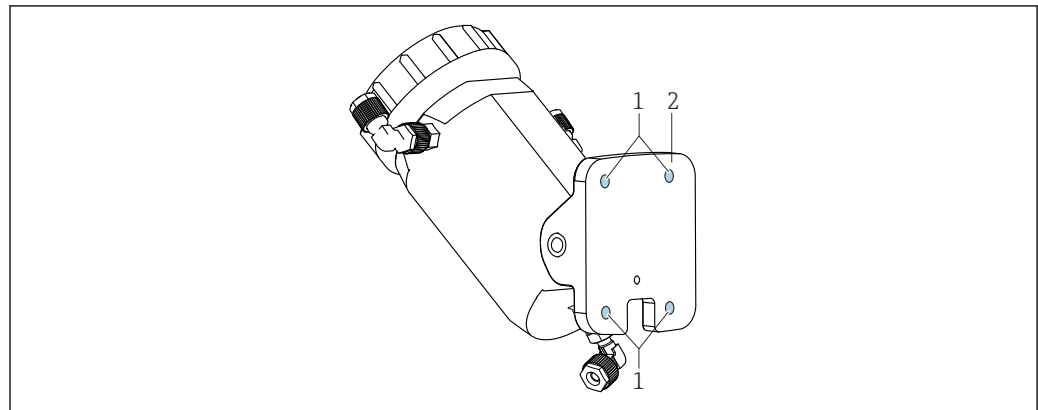
图 14 安装支架后视图
