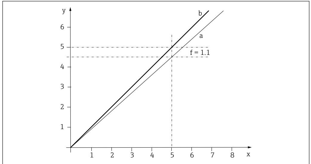
图 27 系数标定原理
