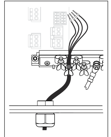
图 21 将电缆安装在接地夹中
