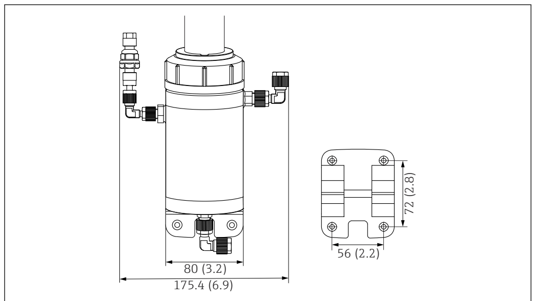
图 4 安装支架带固定板 (右图) 的外形尺寸, 单位: mm (in)
