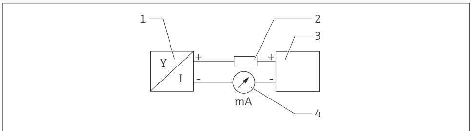
i 1 Blok dijagram HART priključka
