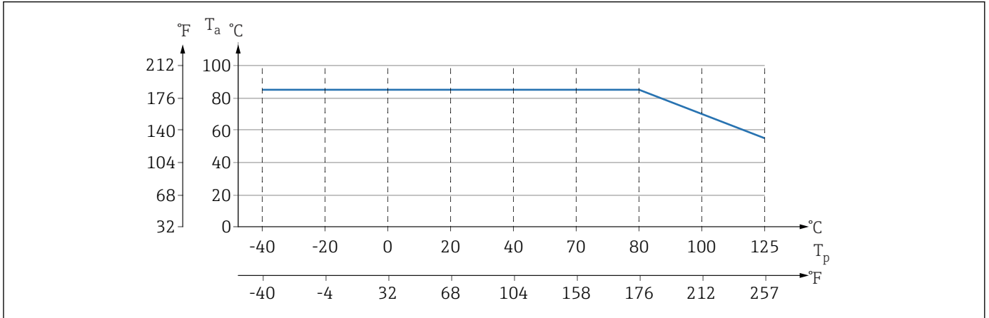
图 7 以上为无保温层垂直安装时的温度范围。
