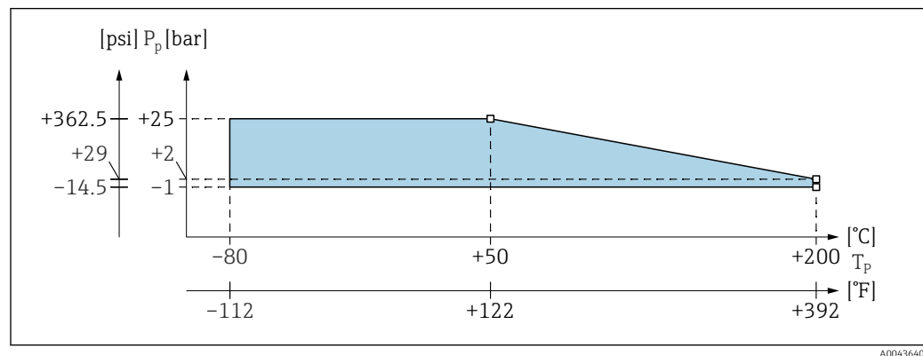
60 Diagramme de déclassement de la pression et de la température pour les sondes à câble sans longueur inactive ou avec longueur inactive
