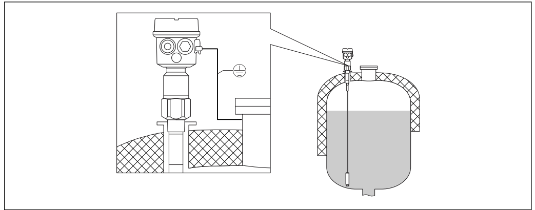
▣ 4 Une sonde avec une longueur inactive pour les cuves isolées
