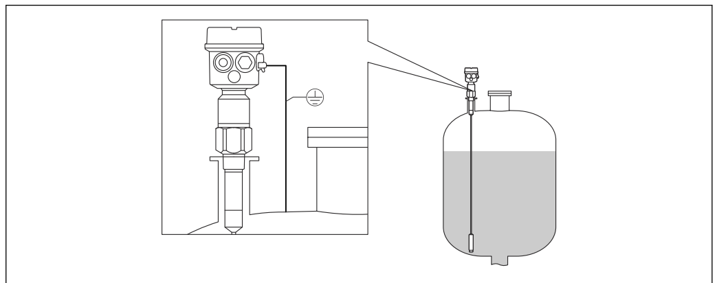
▣ 5 Une sonde avec une longueur inactive entièrement isolée
