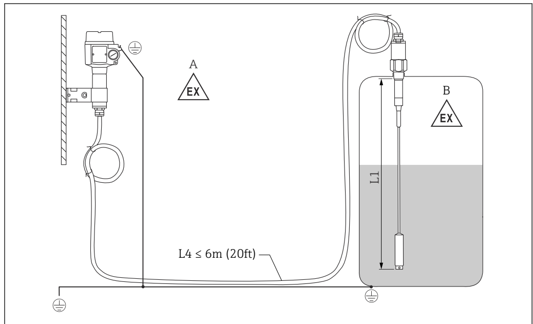
7 Raccordement de la sonde et du boîtier séparé. Unité de mesure mm (in)
