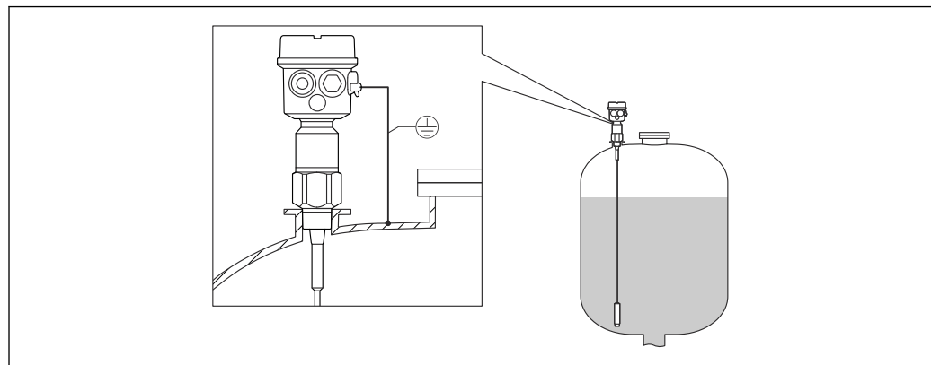
3 Une sonde avec des cuves conductrices
