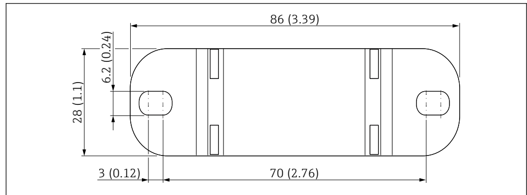
9 Aperçu de support mural. Unité de mesure mm (in)
