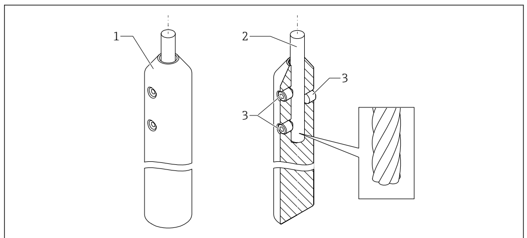
▣ 6 Aperçu du contrepois tenseur
