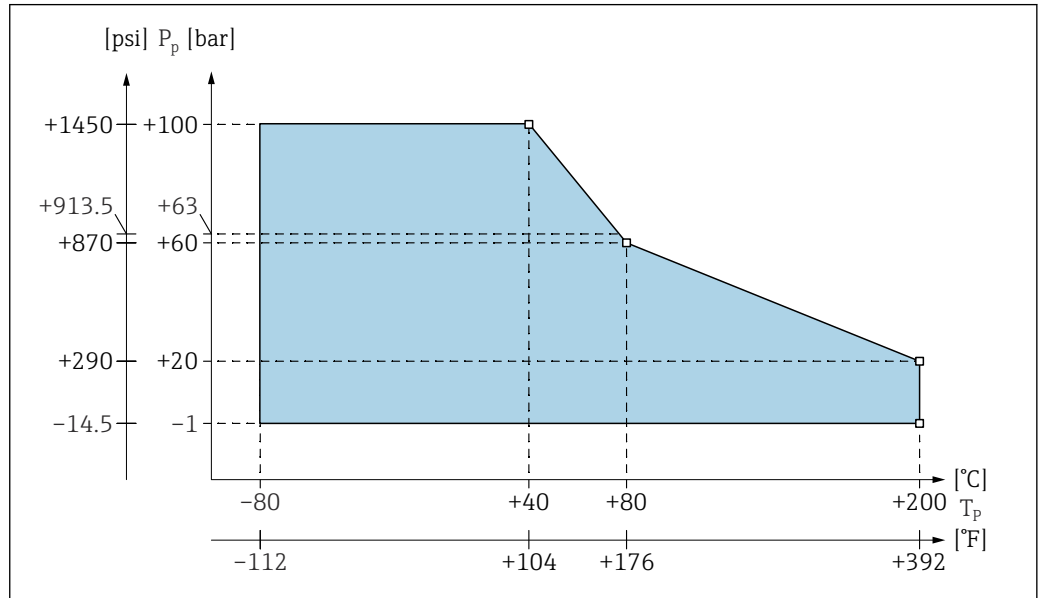
61 Diagramme de déclassement de la pression et de la température pour les sondes à câble sans longueur inactive ou avec longueur inactive
