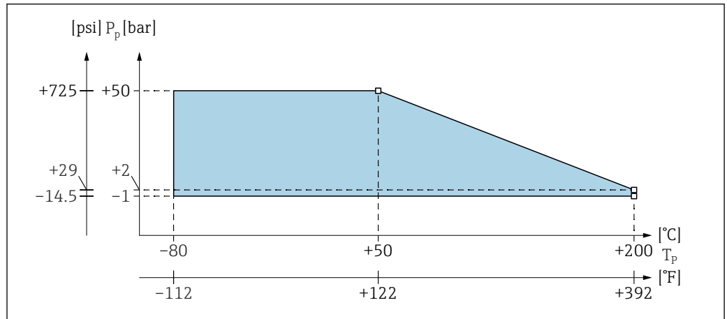
62 Diagramme de déclasserement de la pression et de la température pour les sondes à câble de longueur inactive entièrement isolées
