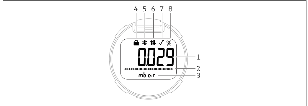
图 10 段码显示屏
