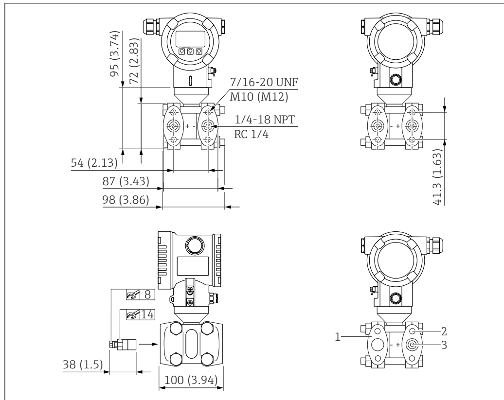
图 8 正视图、左视图、右视图。测量单位 mm (in)
