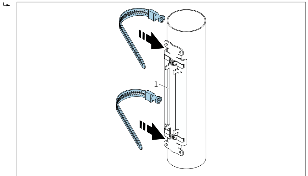
図 23 センサホルダを配置して締付けバンドを取り付けます。
