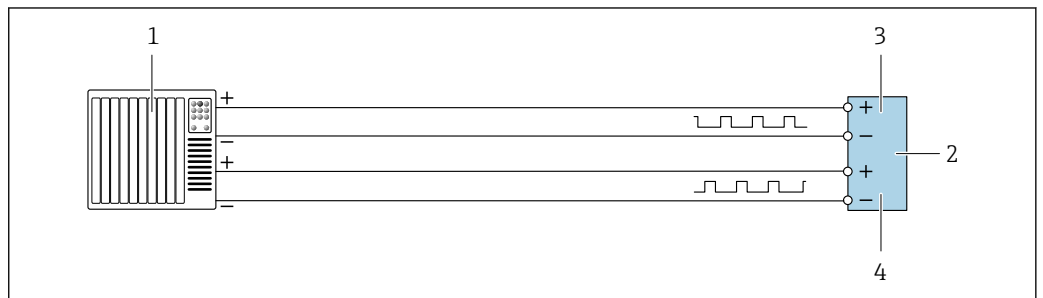
図 53 パルス出力、フェーズシフト（アクティブ）の接続例
