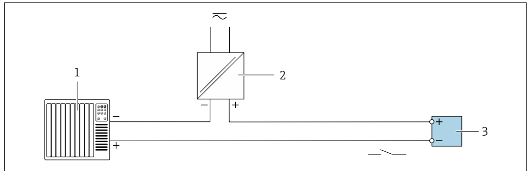
図 52 スイッチ出力（パッシブ）の接続例
