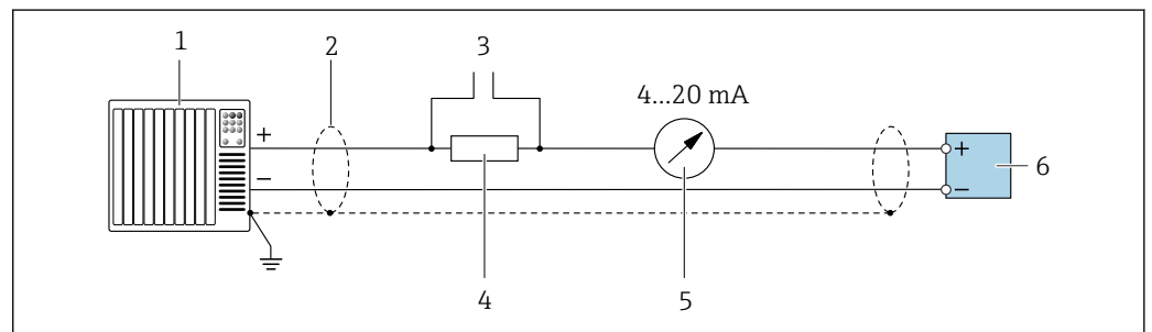
図 46 4~20 mA HART 電流出力 (アクティブ) の接続例
