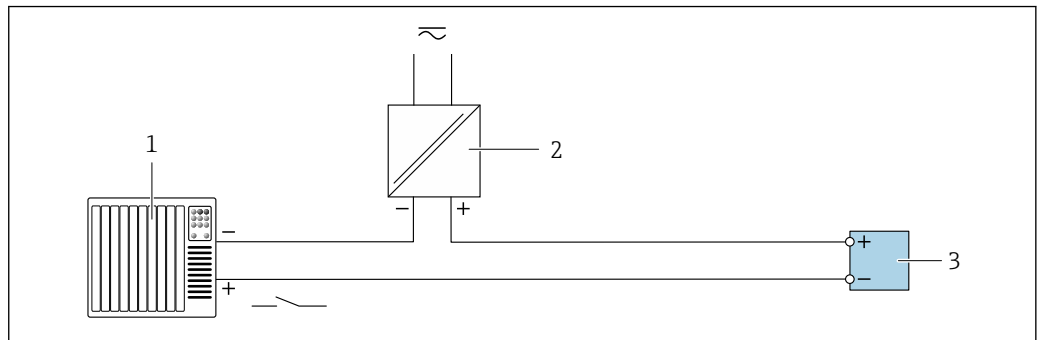
図 57 ステータス入力の接続例
