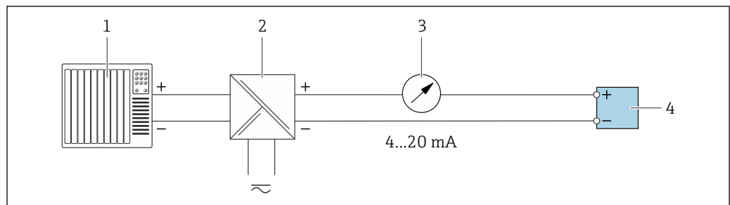
図 50 4~20 mA 電流出力 (パッシブ) の接続例
