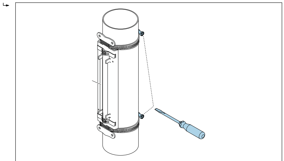
図 24 締付けバンドの締めネジを締め付けます。
