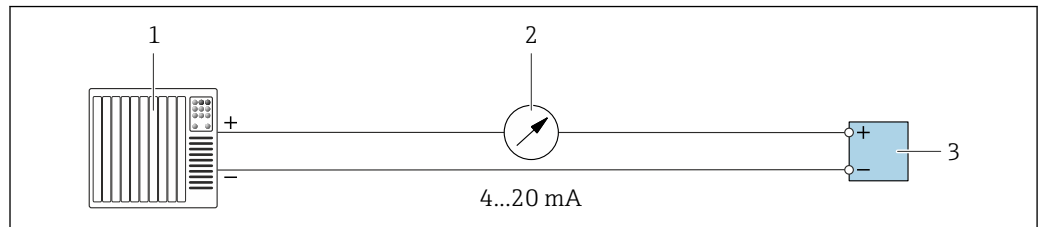
図 49 4~20 mA 電流出力 (アクティブ) の接続例
