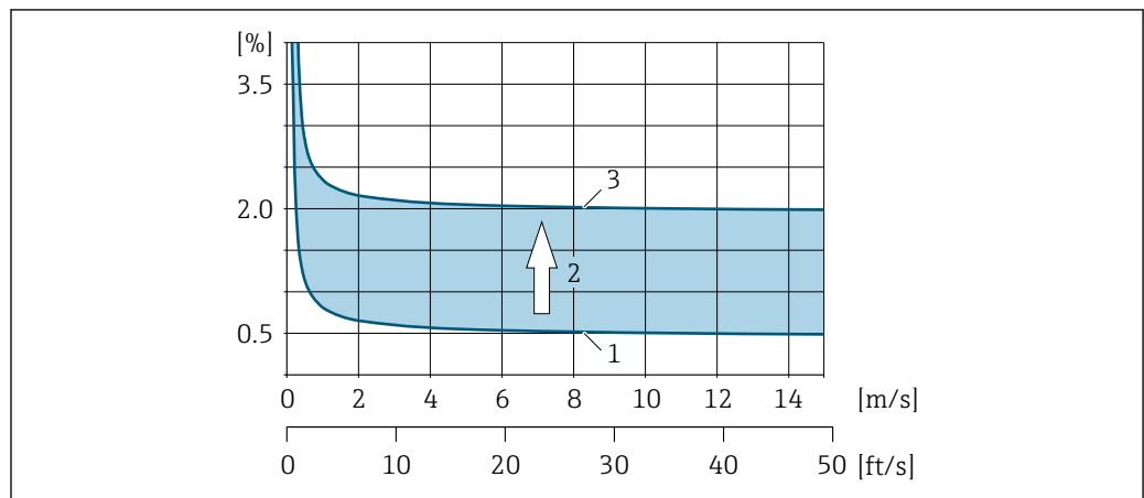
図 73 呼び口径 200A (8") 以上の配管における測定誤差の絶対値の例
