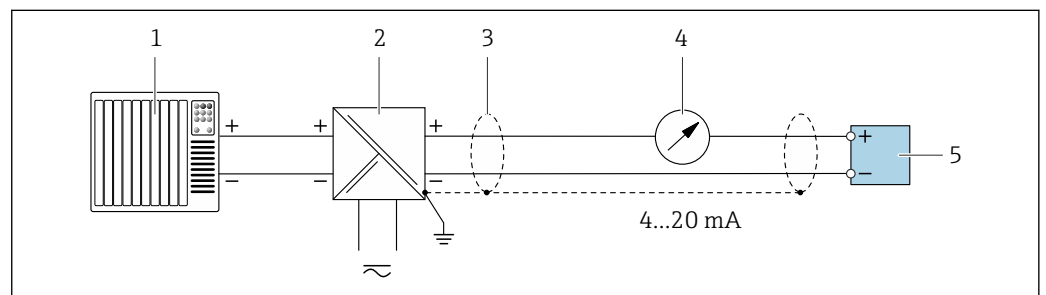
図 47 4~20 mA HART 電流出力 (パッシブ) の接続例
