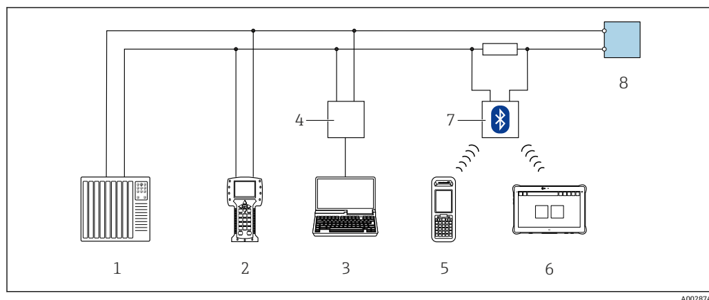
図 62 HART プロトコル経由のリモート操作オプション (アクティブ)
