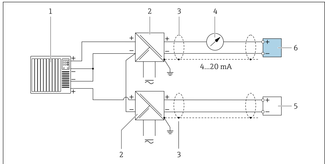
図 48 マイナスコモン HART 入力 (パッシブ) の接続例
