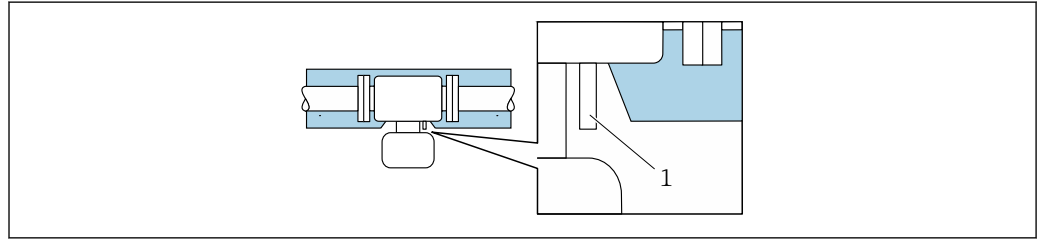
図 36 伸長ネックと圧力測定センサが露出した状態での断熱
