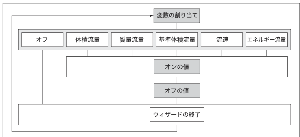
図 31 「設定」メニューの「ローフローカットオフ」ウィザード
