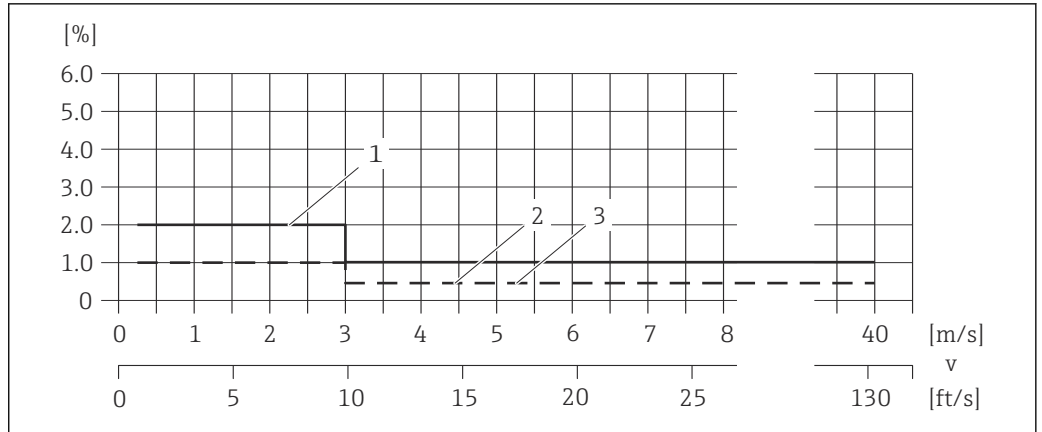
図 35 最大測定誤差 (体積流量)、対読み値 %
