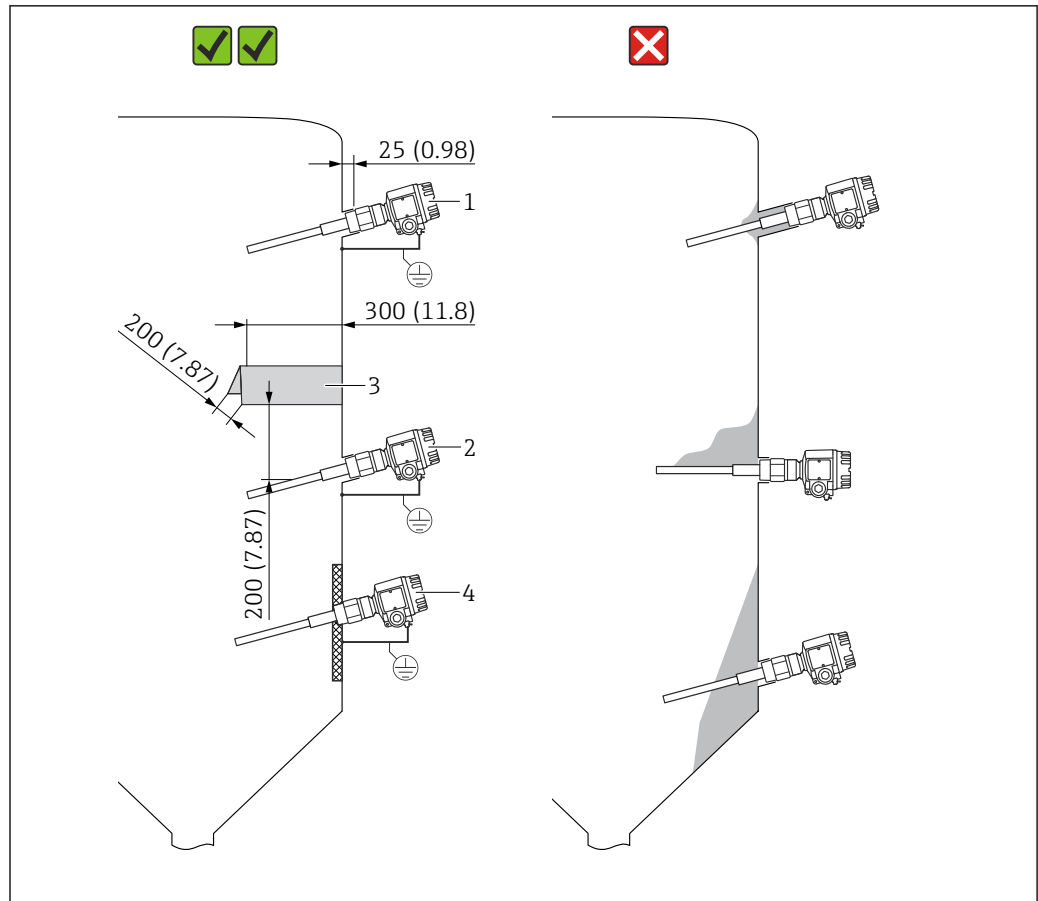
図2 プローブの側面取付け。測定単位 mm (in)
