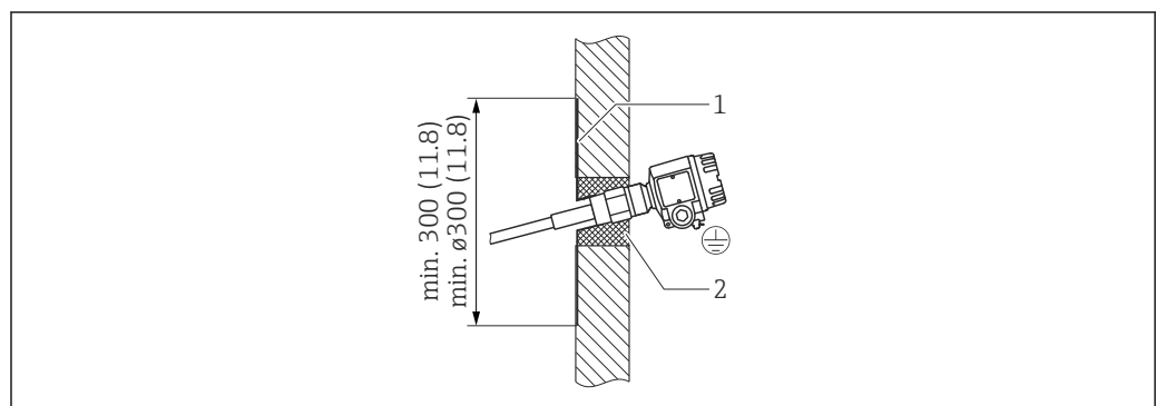
図3 コンクリート壁へのプローブの取付け
