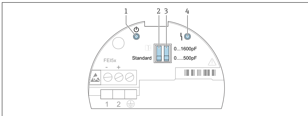
図 19 FEI53 と FEI57S のヒューマンインタフェース
