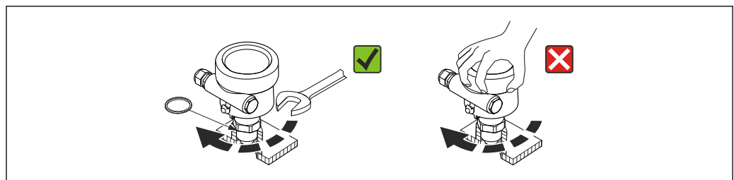
図 7 プローブの正しい設置方法
