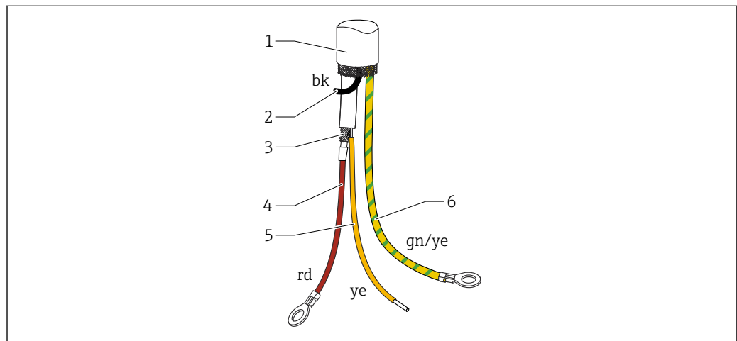
図 12 ケーブル接続部
