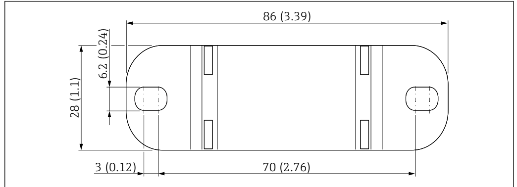
図 10 壁面取付ブラケットの概要。測定単位 mm (in)
