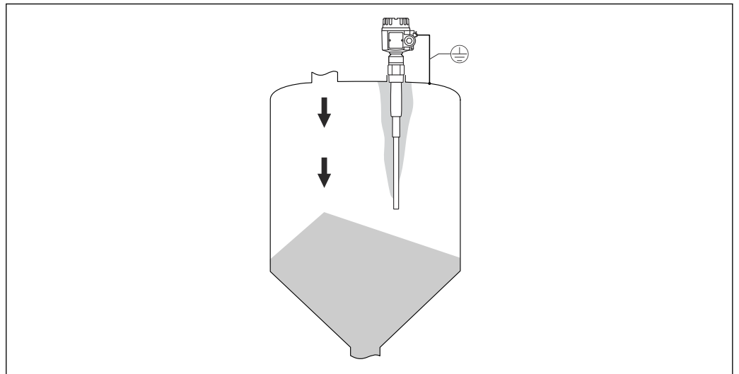
図 5 ロッドプローブ上の付着物
