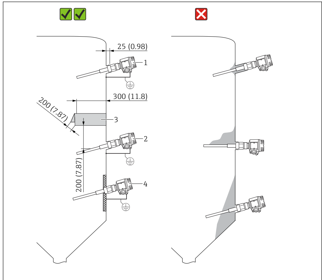
图 2 侧旁安装探头。测量单位 mm (in)
