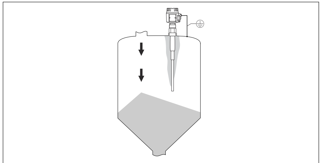
图 5 探杆上存在黏附
