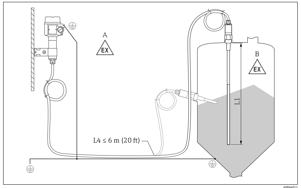
8 连接探头和分离型外壳
