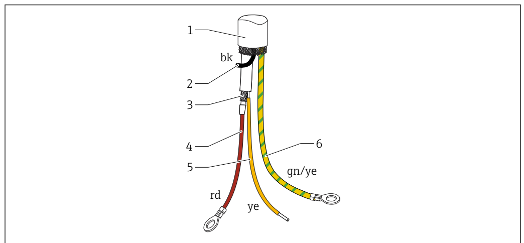
12 电缆的连接线芯
