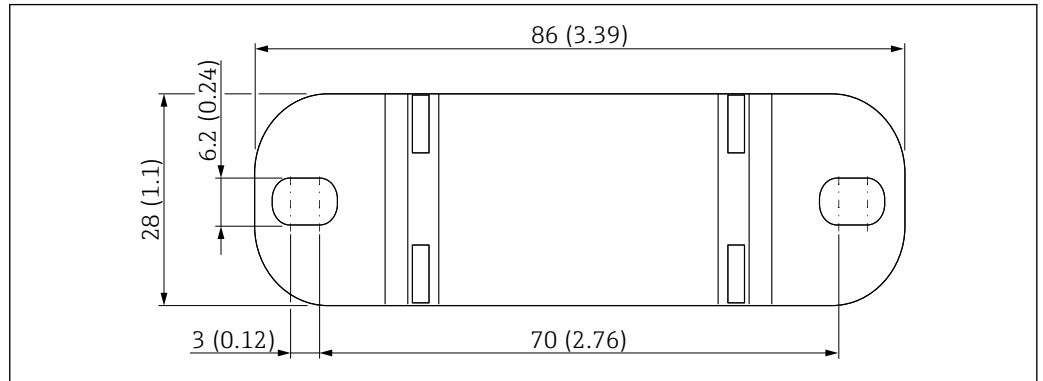
图 10 墙装架示意图。测量单位 mm (in)
