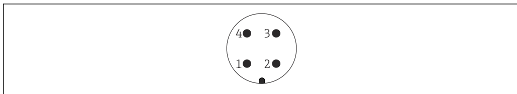
图 15 三线制电子插件 FEI52、FEI53 的 M12 接头
