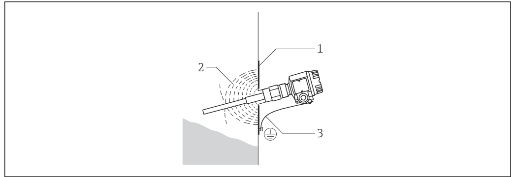
图 4 探头安装在塑料罐壁中
