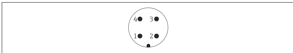
图 14 两线制电子插件 FEI55、FEI57、FEI58、FEI57C 的 M12 接头
