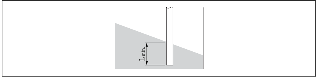
图 6 最小覆盖长度
