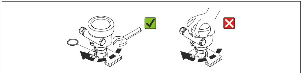
图 7 正确的探头安装方法
