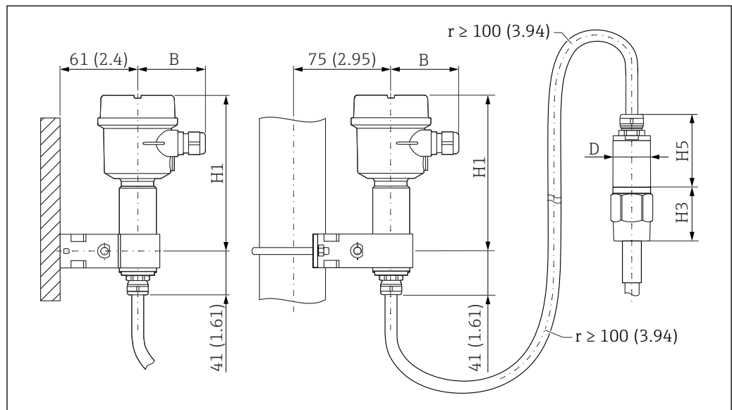
图 9 外壳端（墙装、管装）和传感器端。测量单位 mm (in)
