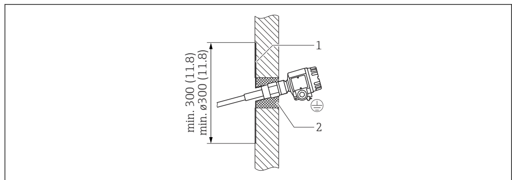
图 3 探头安装在混凝土仓壁中
