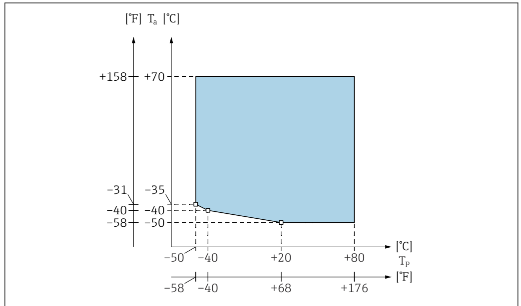
59 Sonde entièrement isolée
