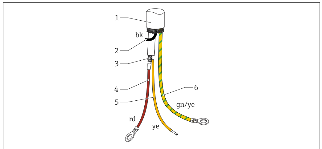
12 Connexions de câble
