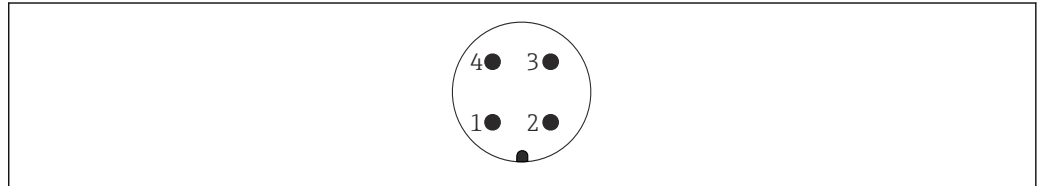
▣ 17 Разъем M12 с 2-проводным подключением электронной вставки FEI55, FEI57, FEI58, FEI57C
