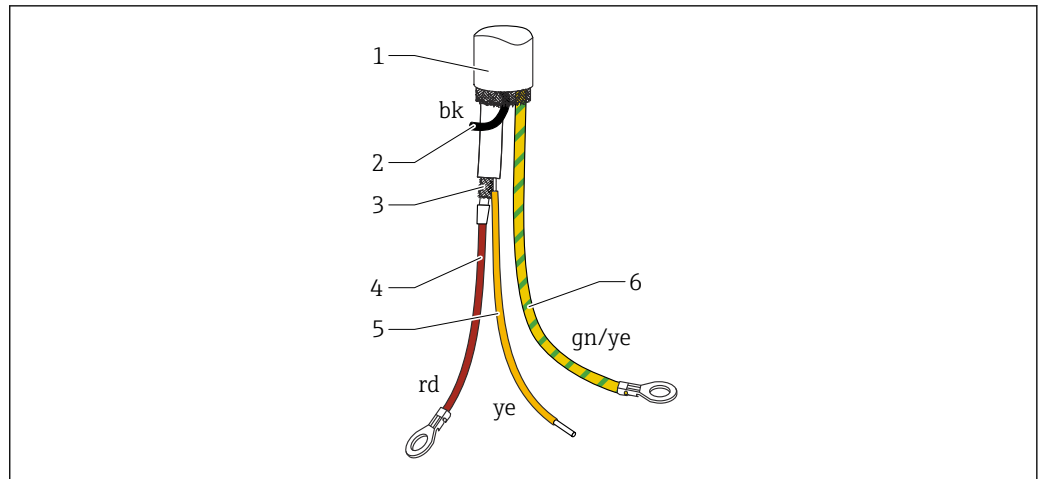
15 Кабельные соединения
