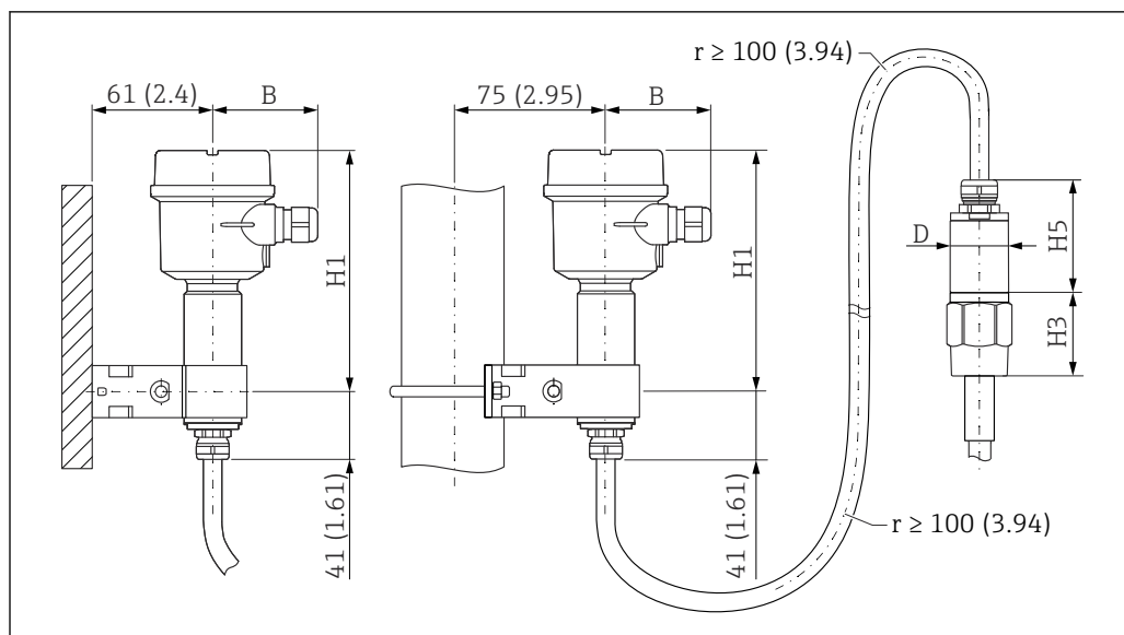
12 Сторона корпуса: настенный монтаж, монтаж на трубопроводе, сторона датчика. Единица измерения мм (дюйм)
