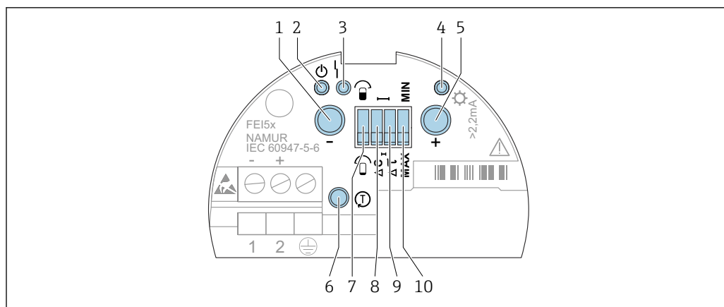
45 Интерфейс пользователя для электронной вставки FEI58
