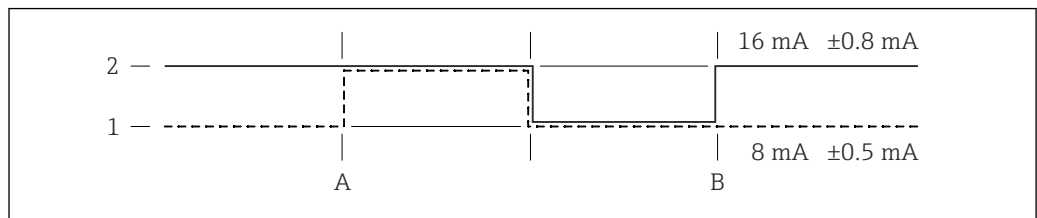
39 Исходная точка: зонд не покрыт
