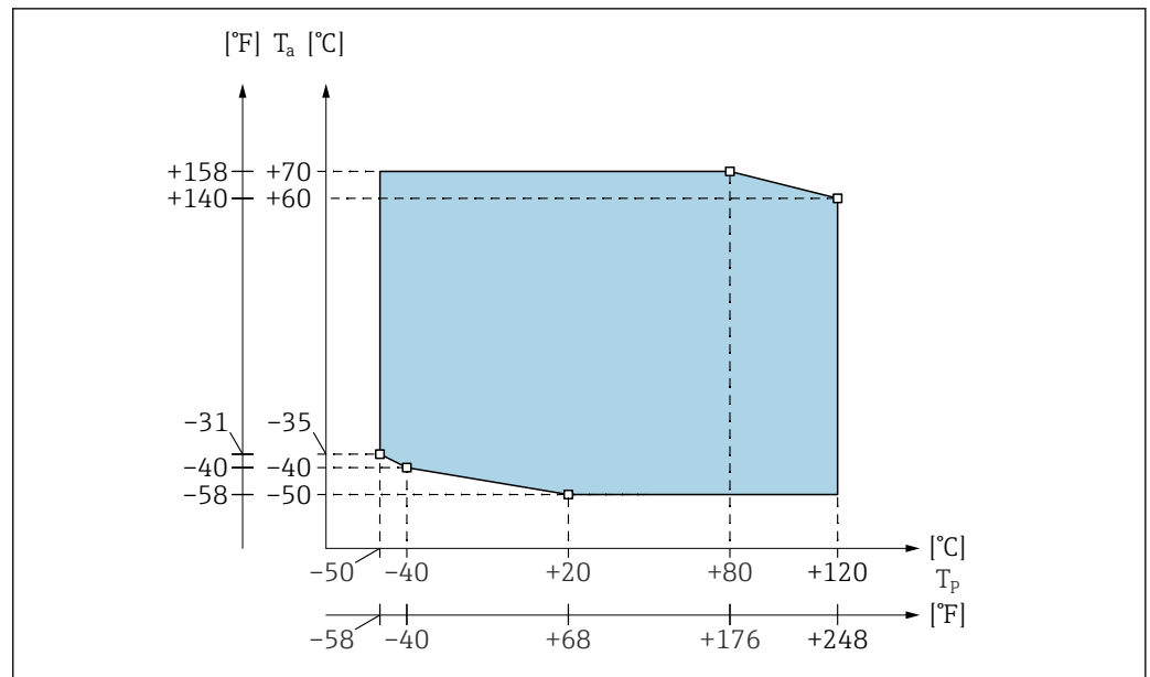
62 Диаграмма диапазона рабочей температуры: полностью изолированный зонд
