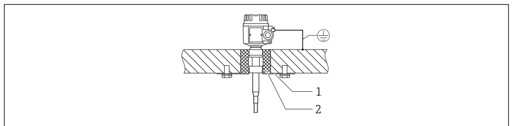
5 Установка на бетонной стенке силоса в случае конденсации
