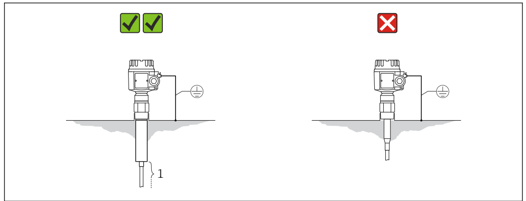
3 Силос со стенками, которые проводят электричество
