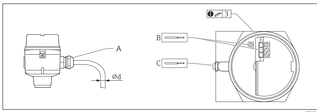
16 Подключение зонда и электронной вставки
