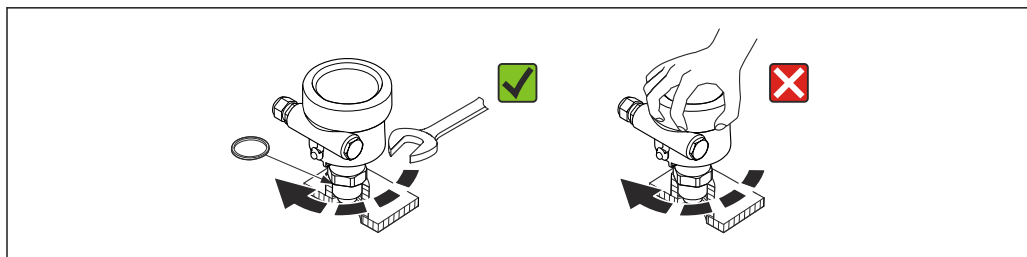
10 Правильный монтаж зонда
