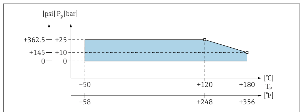
63 Диаграмма отклонения рабочего давления и температуры от номинальных значений: частично изолированный зонд
