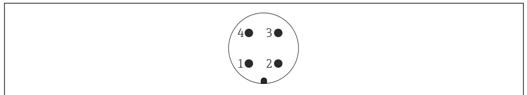
▣ 18 Разъем M12 с 3-проводным подключением электронной вставки FEI52, FEI53
