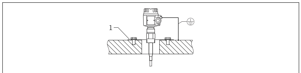
4 Установка на бетонной стенке силоса
