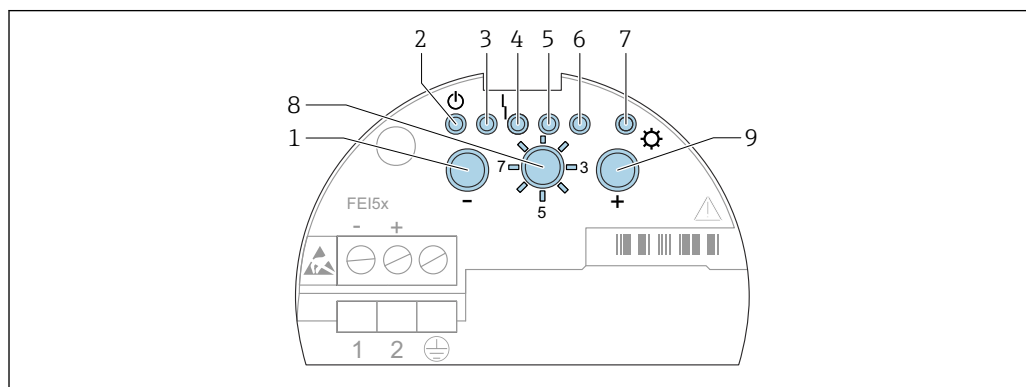
21 Интерфейс пользователя для электронных вставок FEI51, FEI52, FEI54, FEI55
