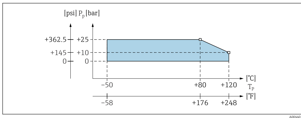
64 Диаграмма отклонения рабочего давления и температуры от номинальных значений: полностью изолированный зонд
