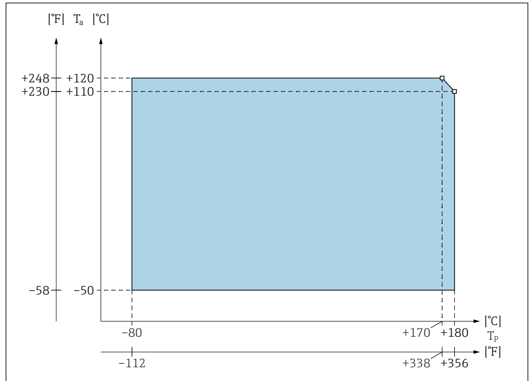
65 Диаграмма диапазона рабочего давления
