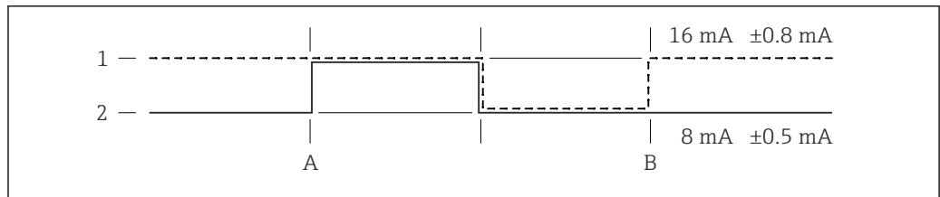
38 Исходная точка: зонд покрыт
