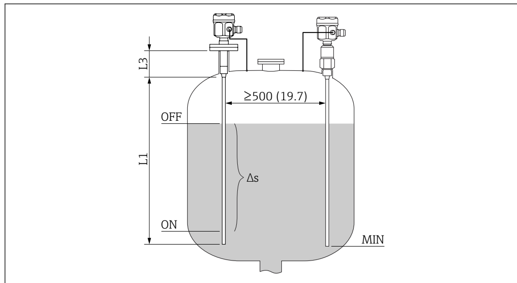
8 Condition de mesure. Unité de mesure mm (in)
