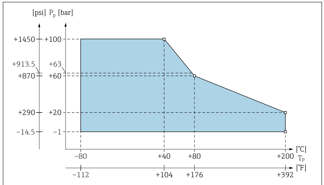
19 Diagramme de déclassement de la pression et de la température de process
