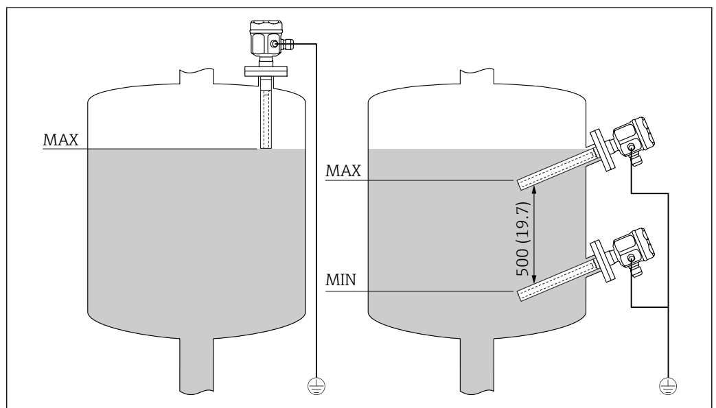
12 Montage du capteur dans des cuves non conductrices. Unité de mesure mm (in)
