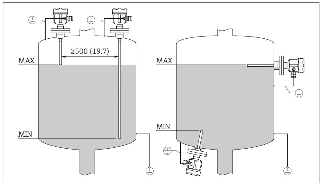
11 Montage du capteur dans des cuves conductrices. Unité de mesure mm (in)
