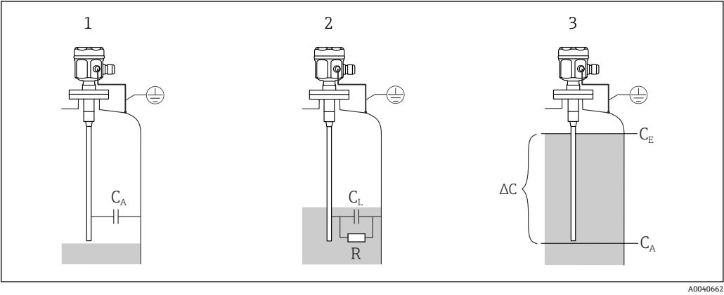
图 1 电容限位检测的测量原理
